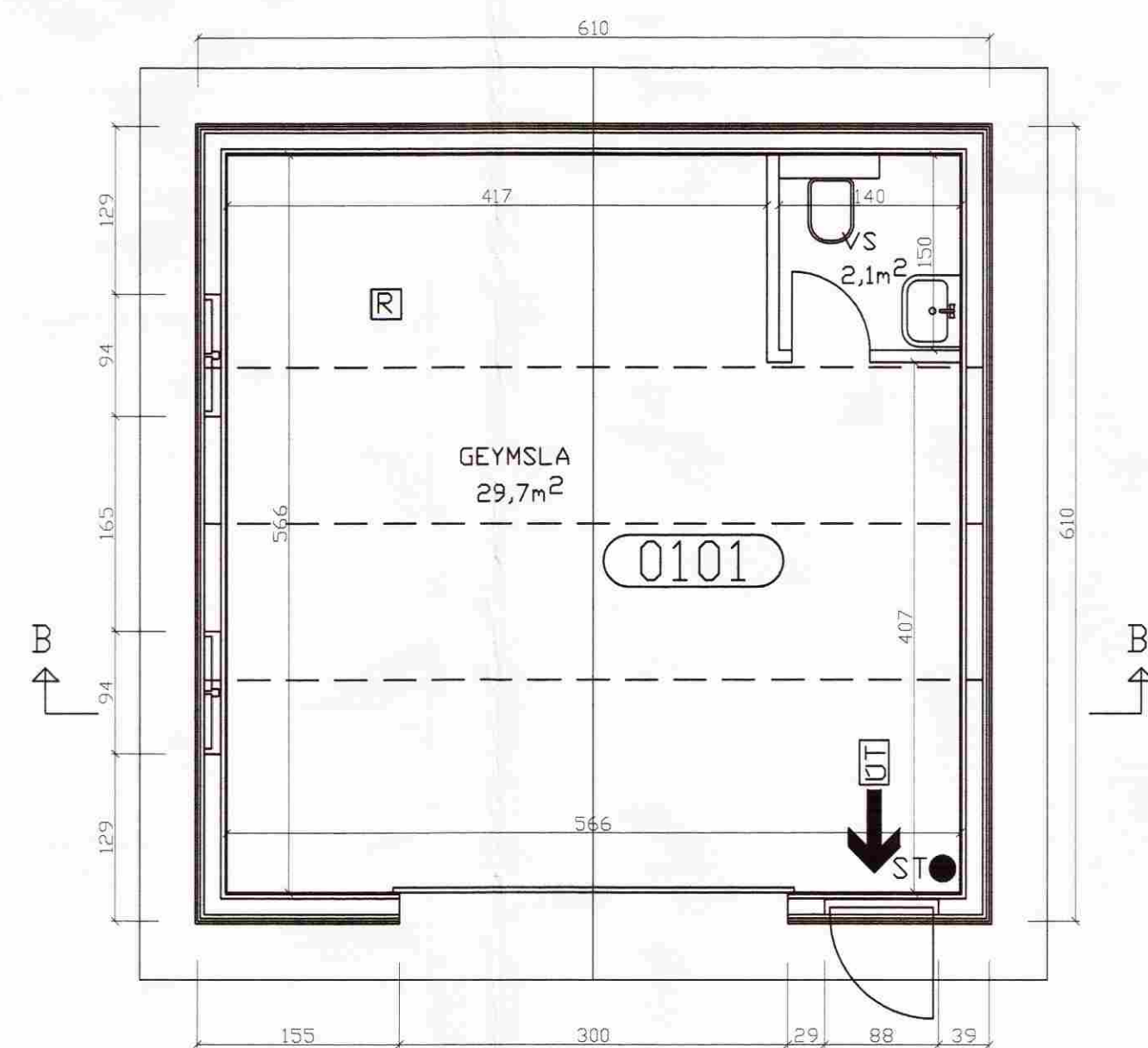
GRUNNMYND
