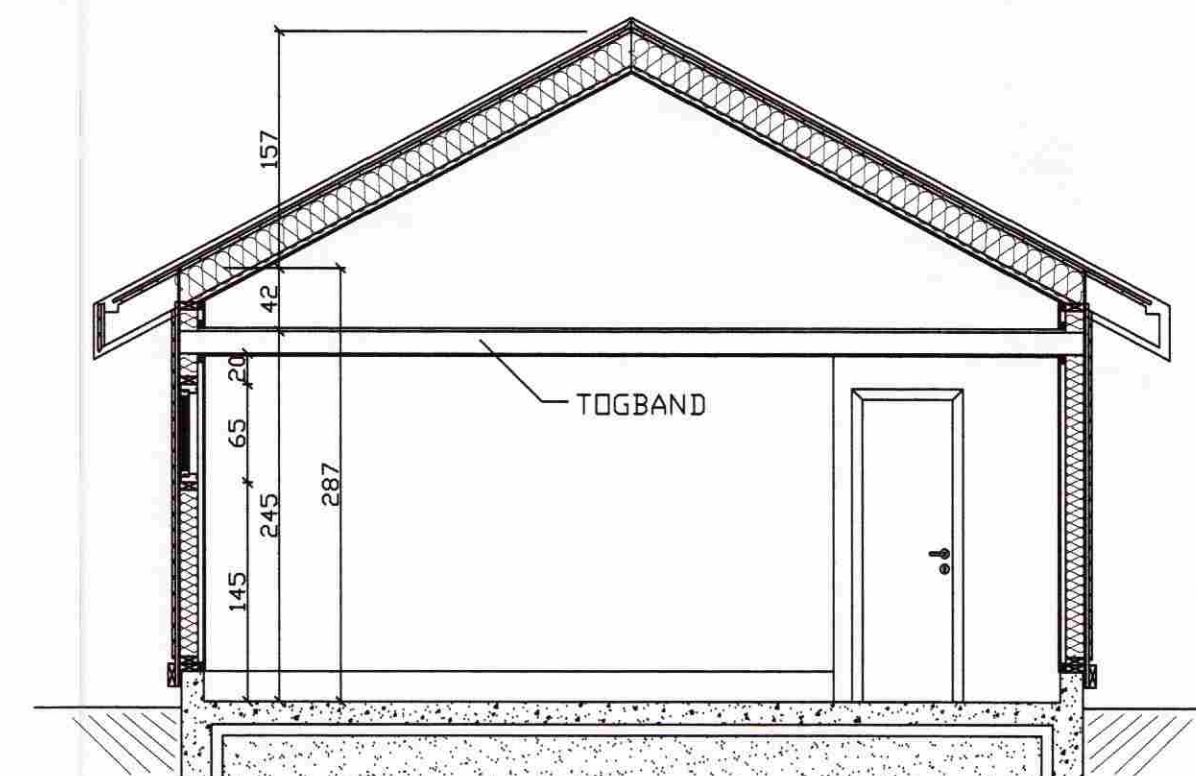
SNIÐ B-B
