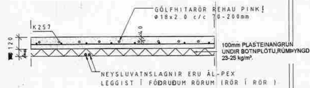
ALMENNT SNID Í BOTNPLÖTU 1:20
