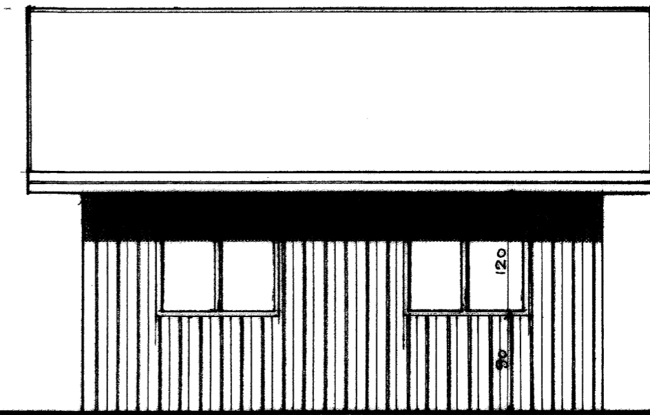
AUSTUR ÚTLIT VERKFERAGEYMSLU
