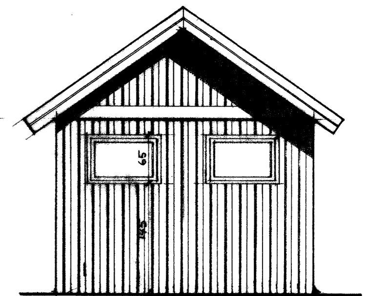
NORÐUR ÚTLIT GEYMSLU
