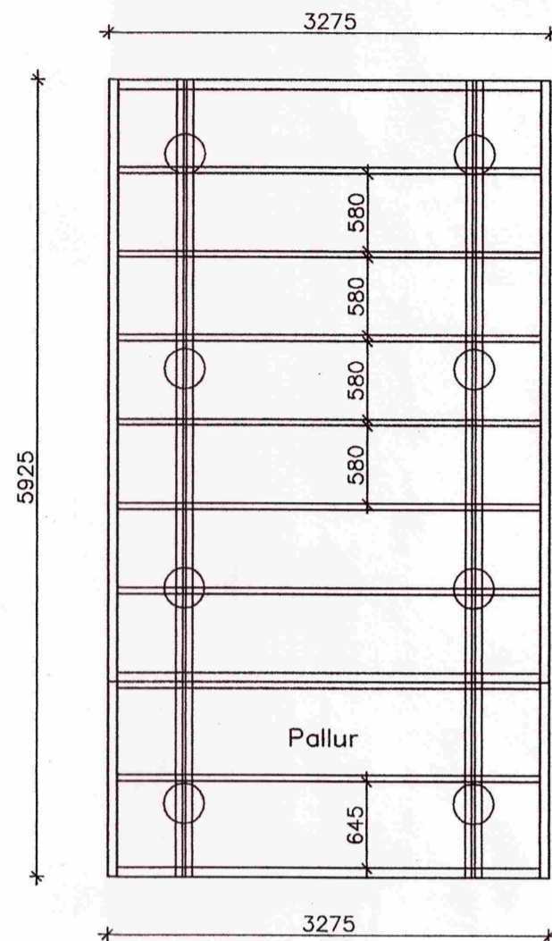
Grunnmynd dregarar
