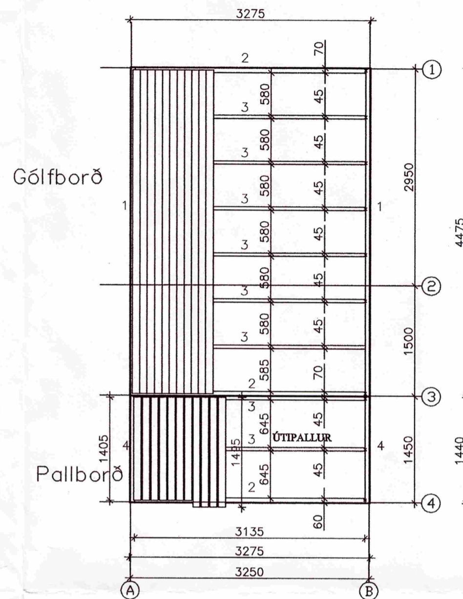
Grunnmynd gólfborð
