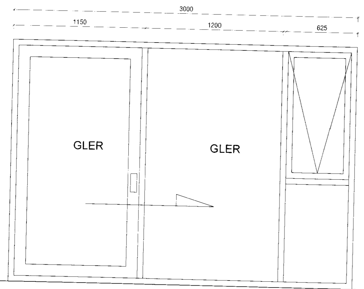
H4: 1 STK OPNUN: RENNIHURÐ
