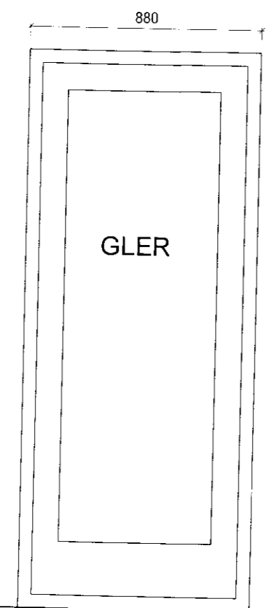
H2: 2 STK OPNUN: HÆGRI ÚT VINSTRI ÚT
