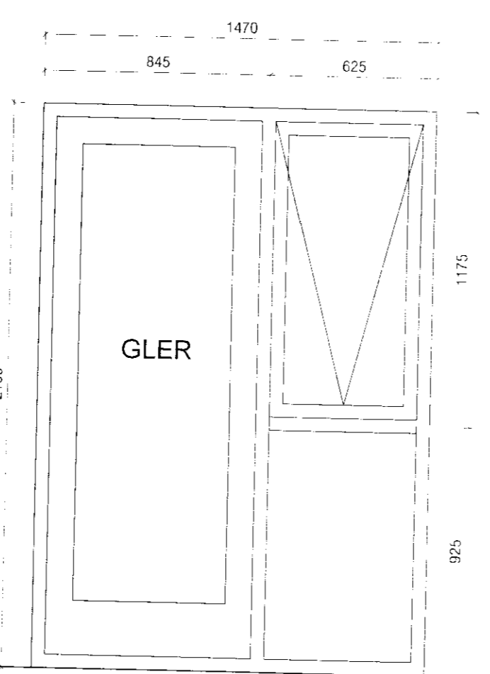
H5: 1 STK OPNUN: HÆGRI ÚT
