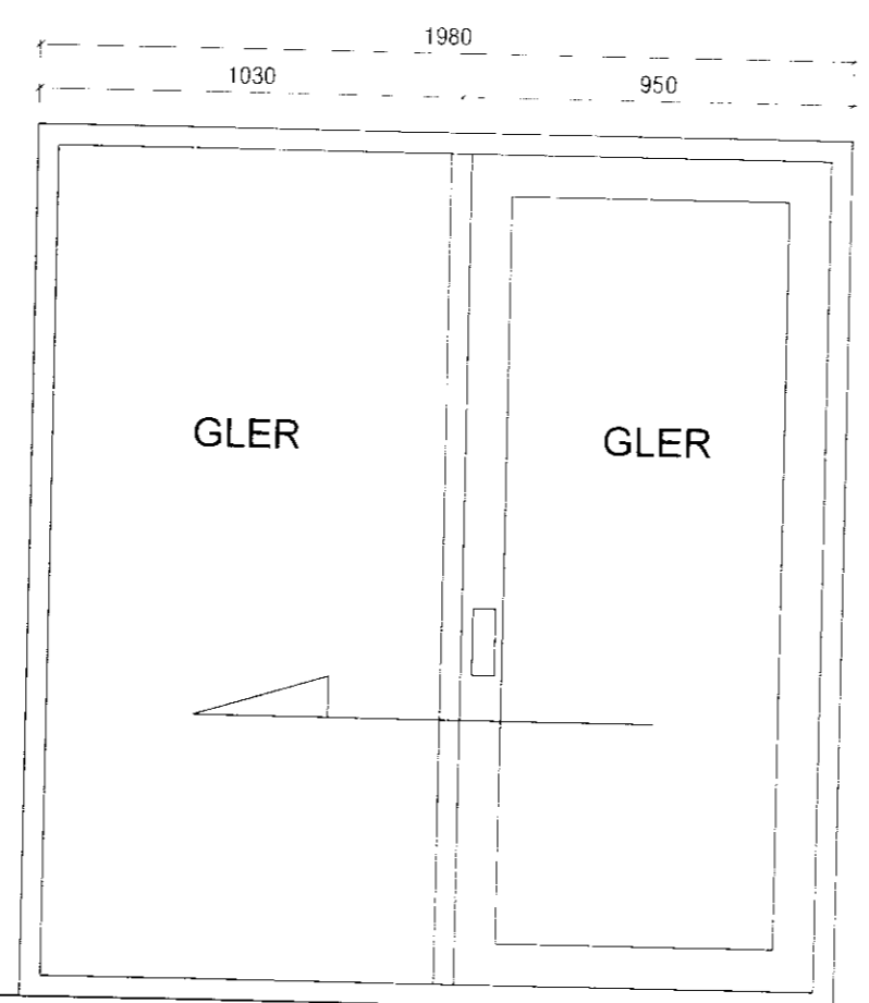
H3: 1 STK OPNUN: RENNIHURÐ
