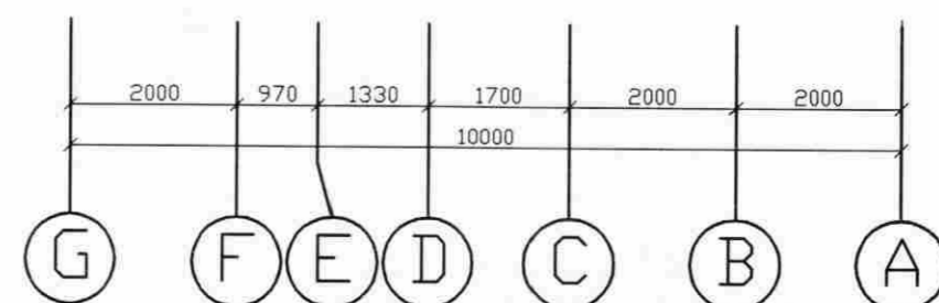
ÚTLIT SUDURHLID
