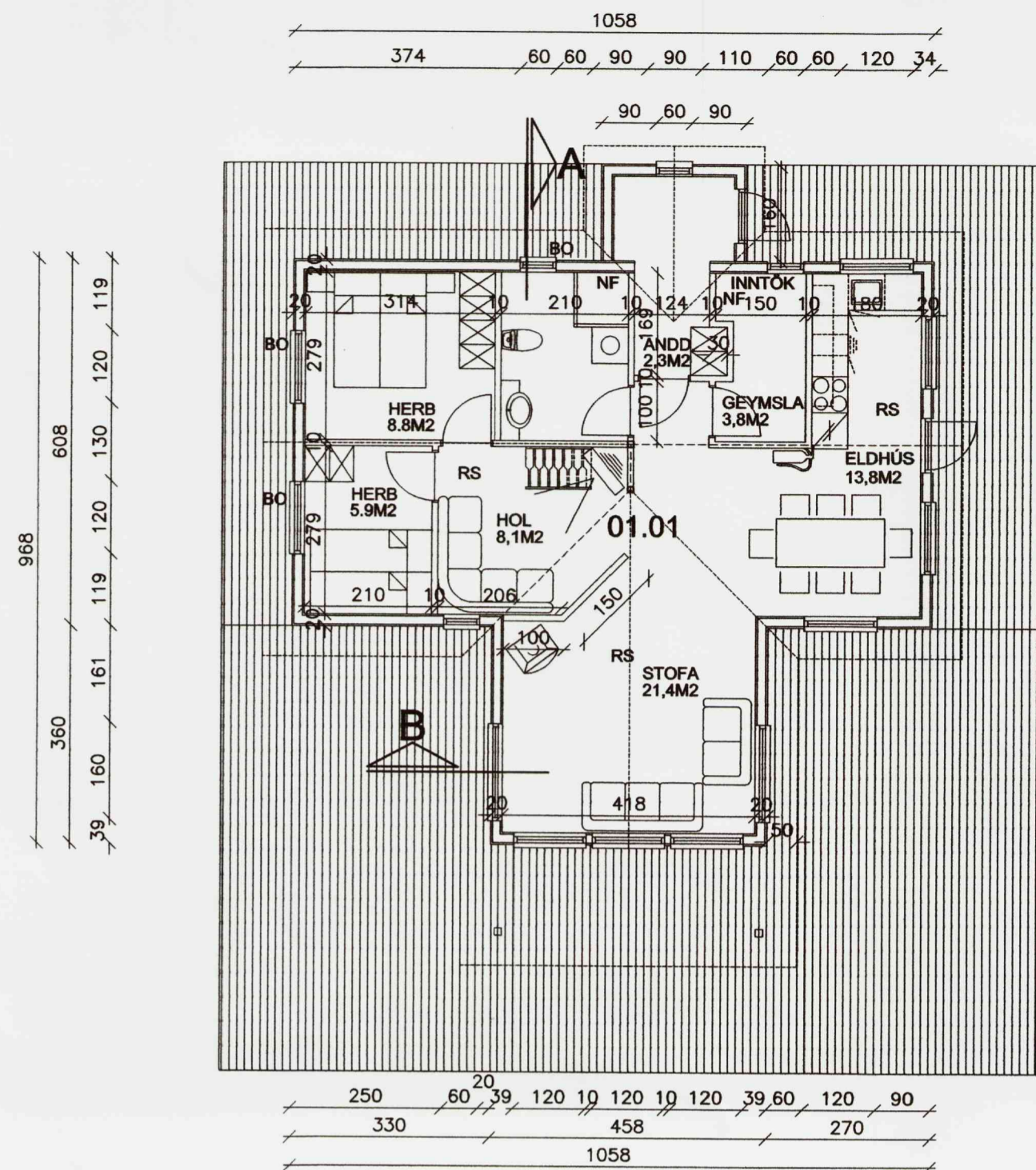
GRUNNMYND JARÐHÆÐ
