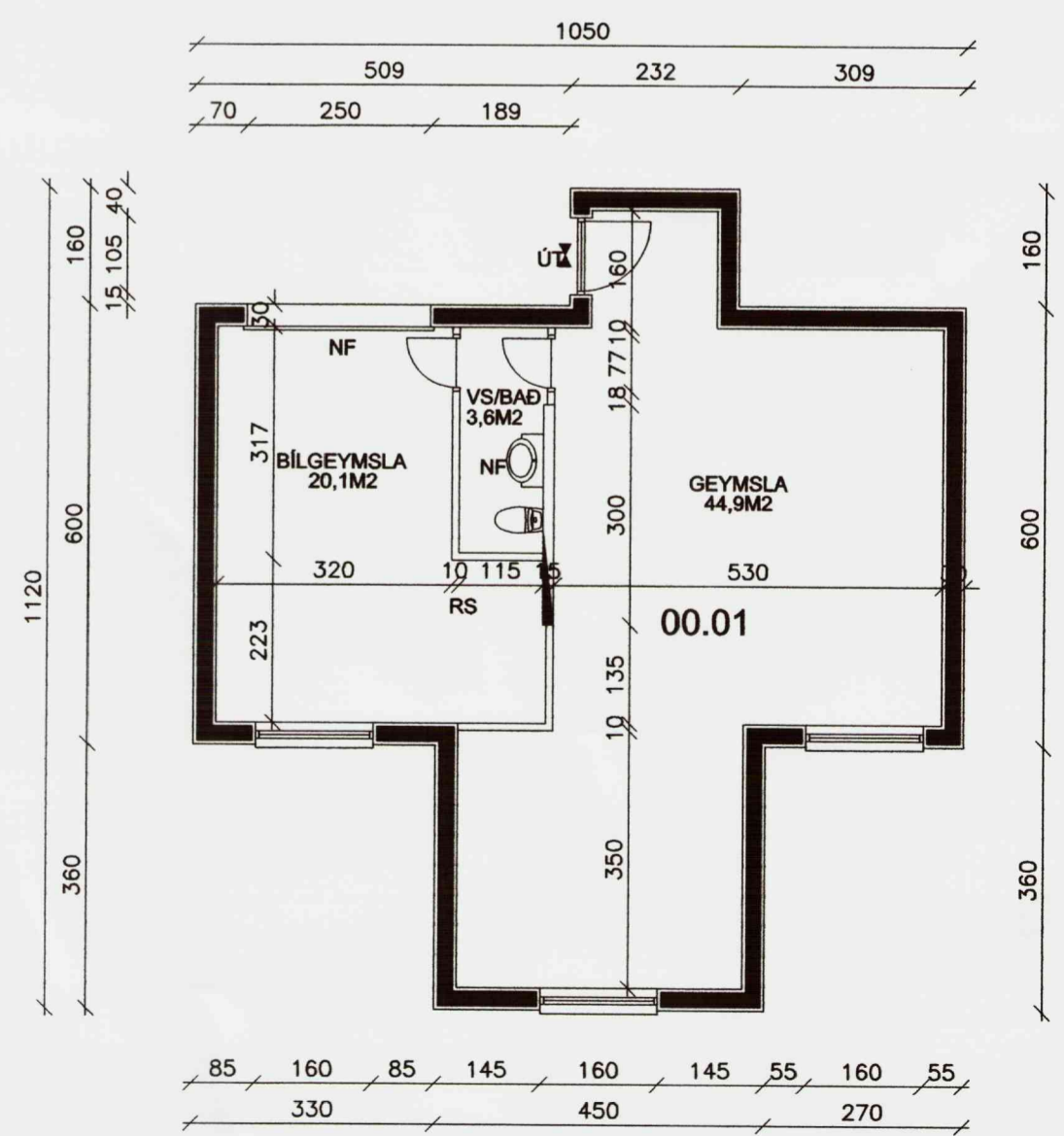
GRUNNMYND KJALLARI
