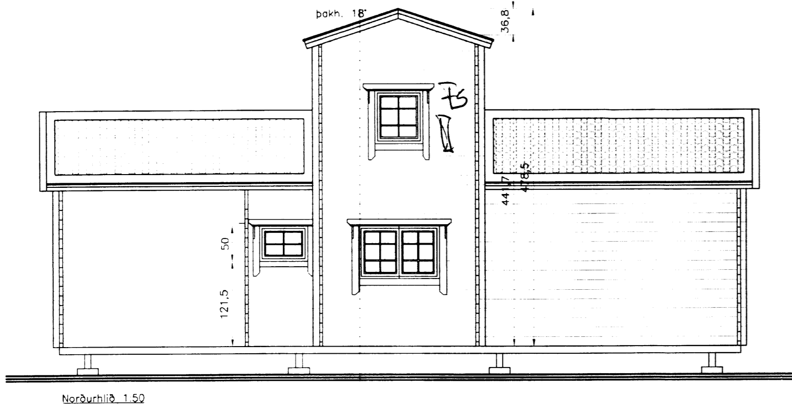
Norðurhlíð 1:50
