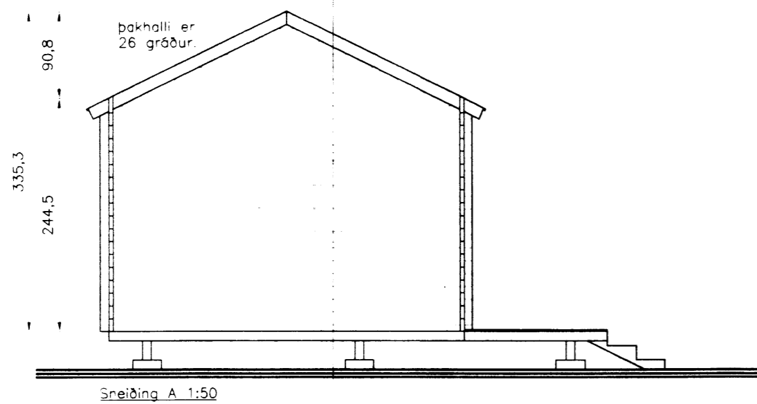
Sneiðing A 1:50
