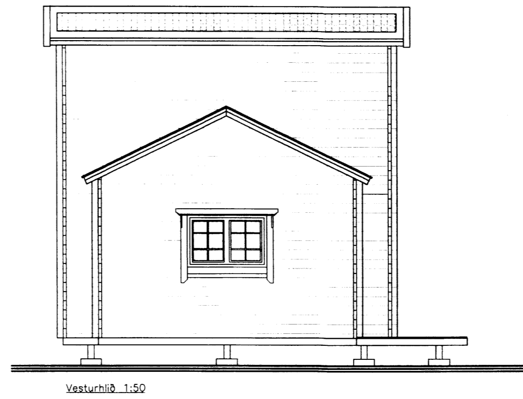
Vesturhlíð 1:50
