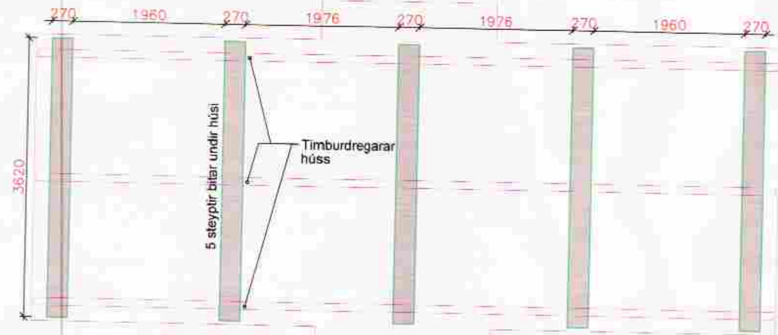
Grunnmynd undirstaða
