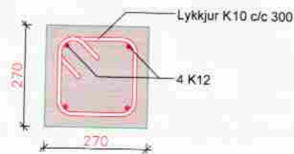
Steiptur biti Þversnið 1:10
