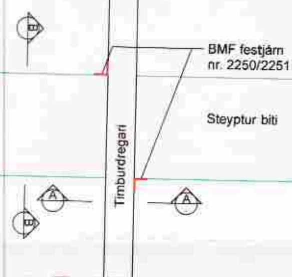
Samskeyti bita og dregara Grunnmynd 1:10
