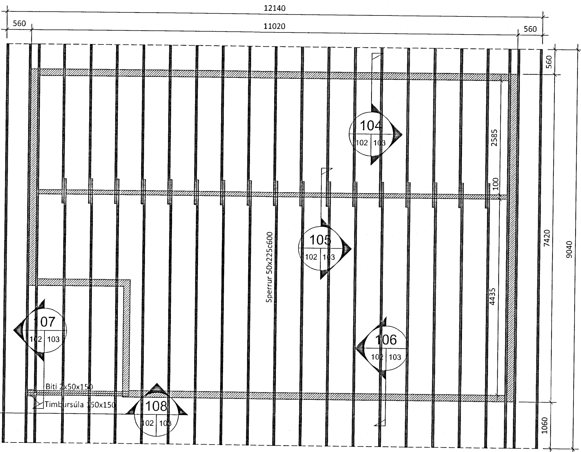
GRUNNMYND-ÞAKVIRKI Mkv. 1:50
