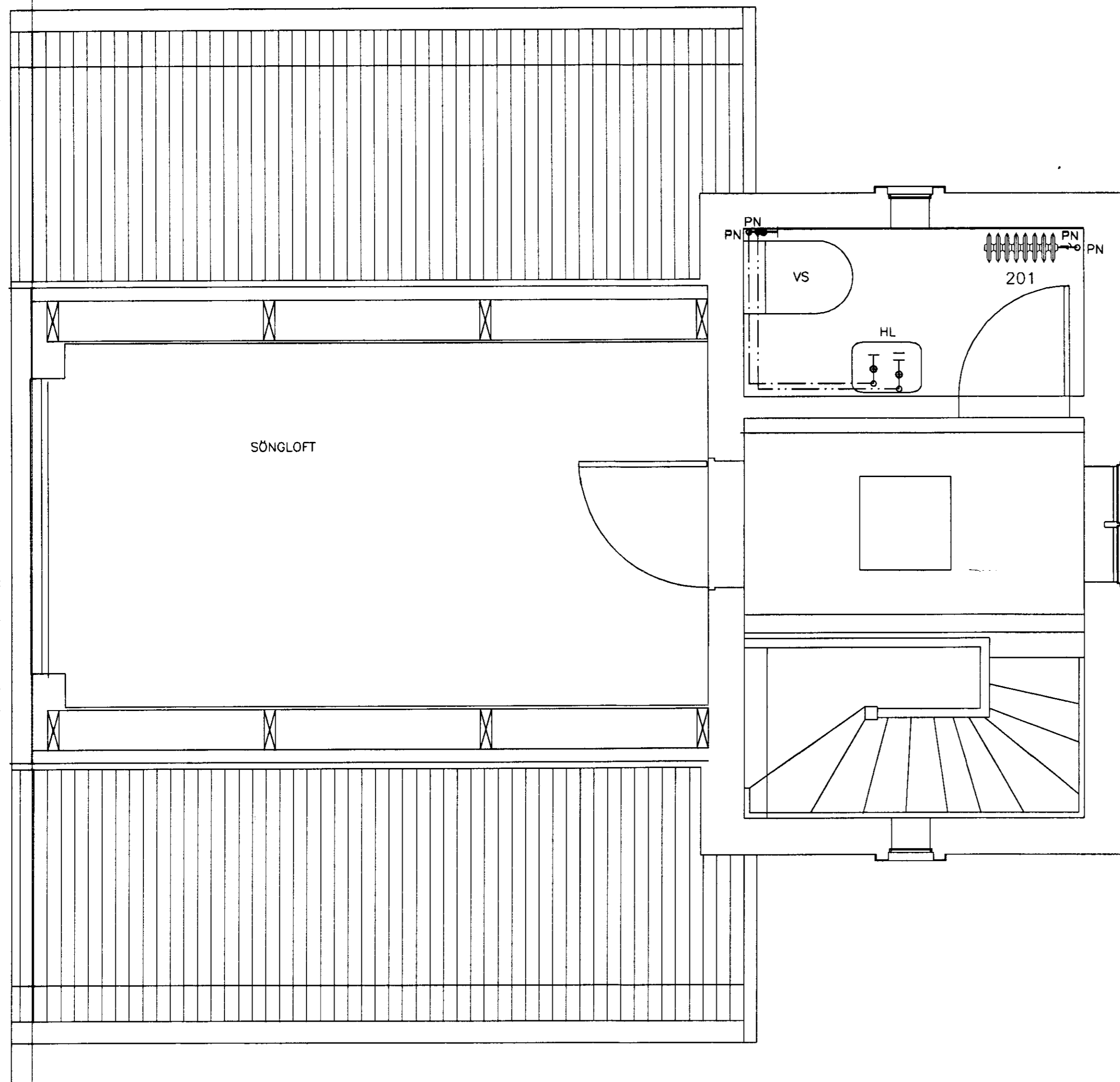
GRUNNMYND 2. HÆÐ
