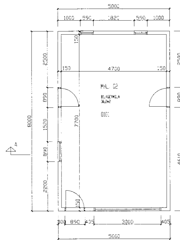
GRUNNMYND
