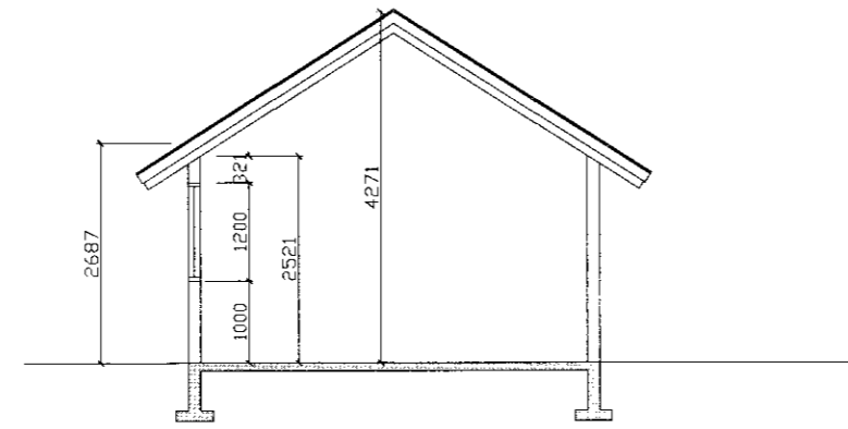
SNID A-A
