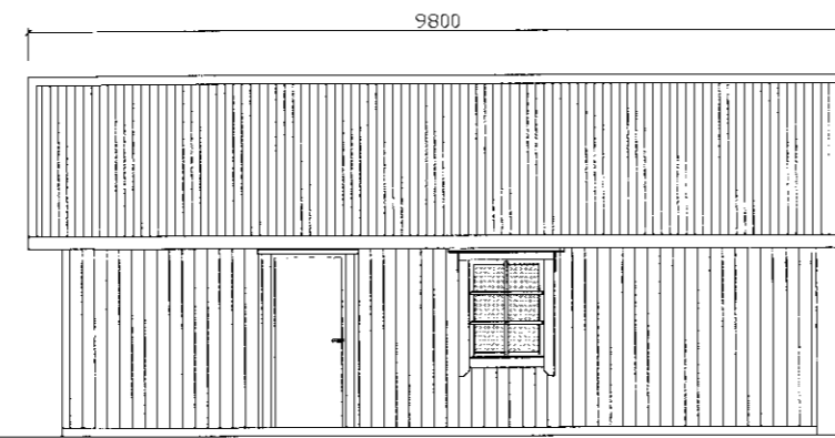
ÚTLIT SUÐUR
