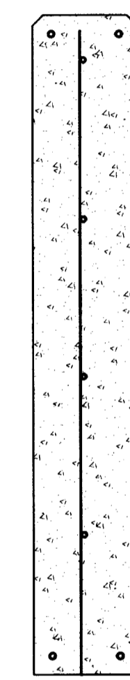
SÖKKULL, ÞVERSNIÐ
