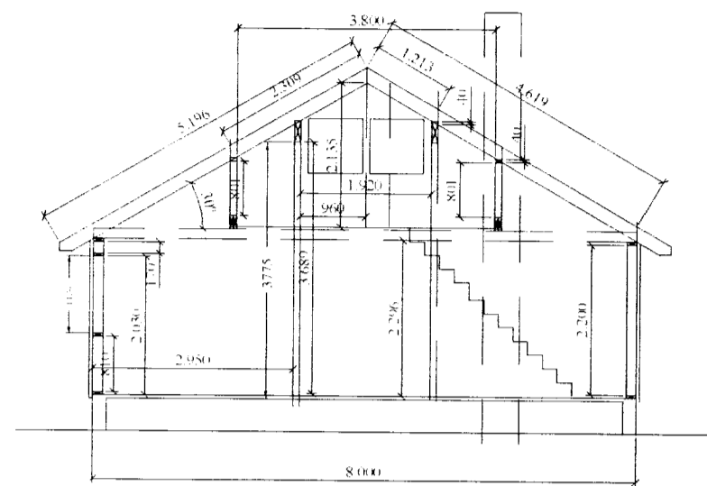
Snið A-A
