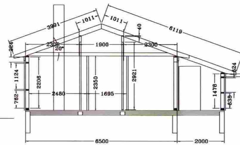
SNID A-A
