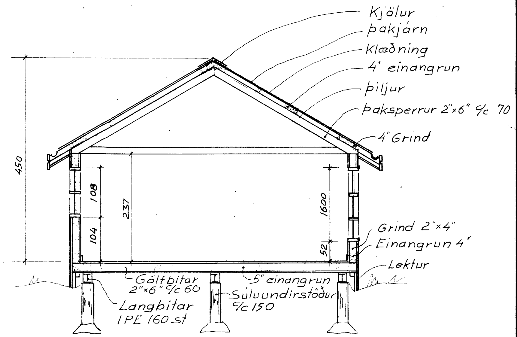
Snið A-A
