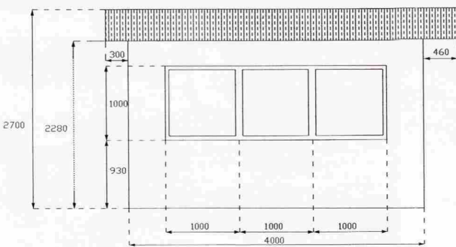
Suð-austur Mkv.1:50
