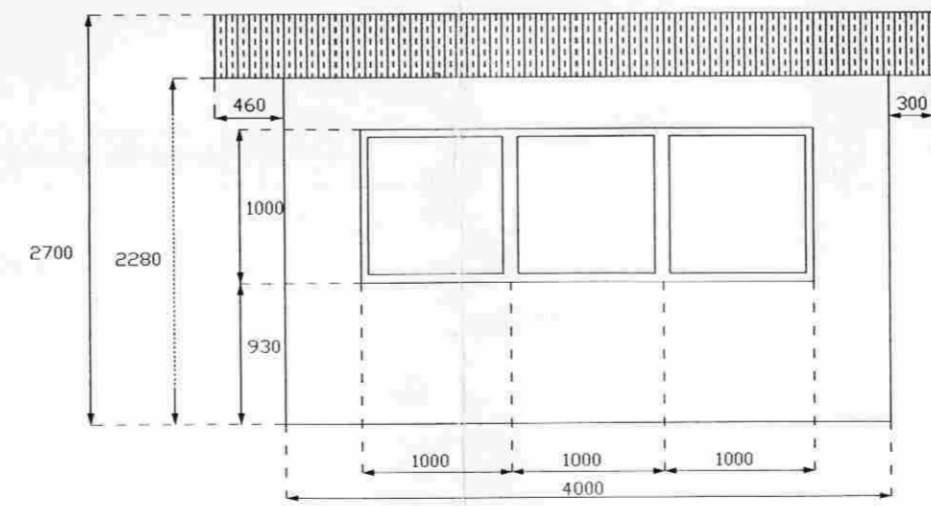
Norð-vestur Mkv.1:50
