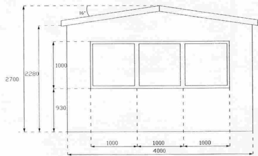
Suð-vestur Mkv.1:50
