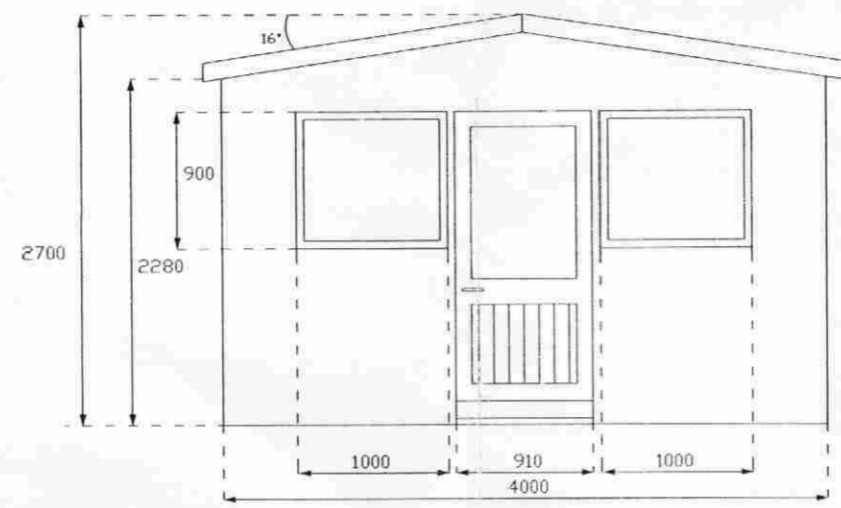
Norð-austur Mkv.1:50
