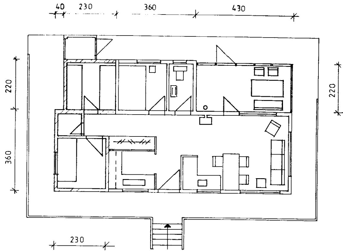
GRUNNMYND 1:100
