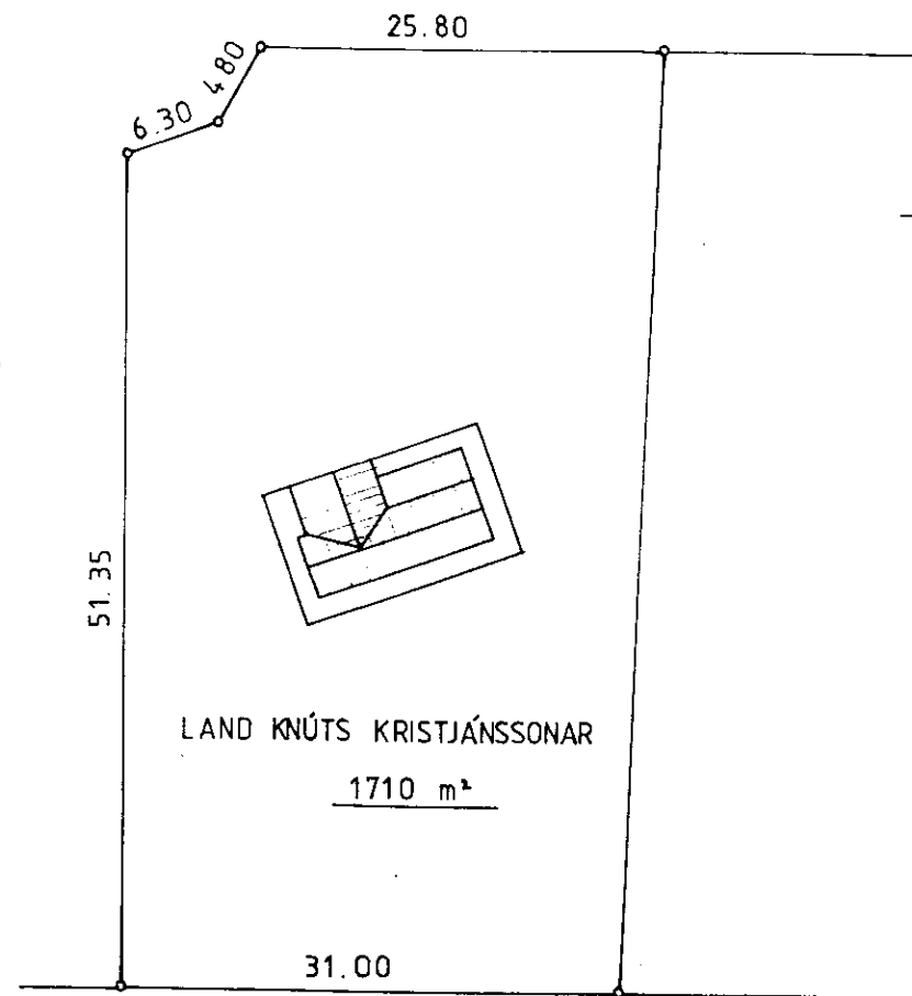
AFSTÖÐUMYND 1:500
