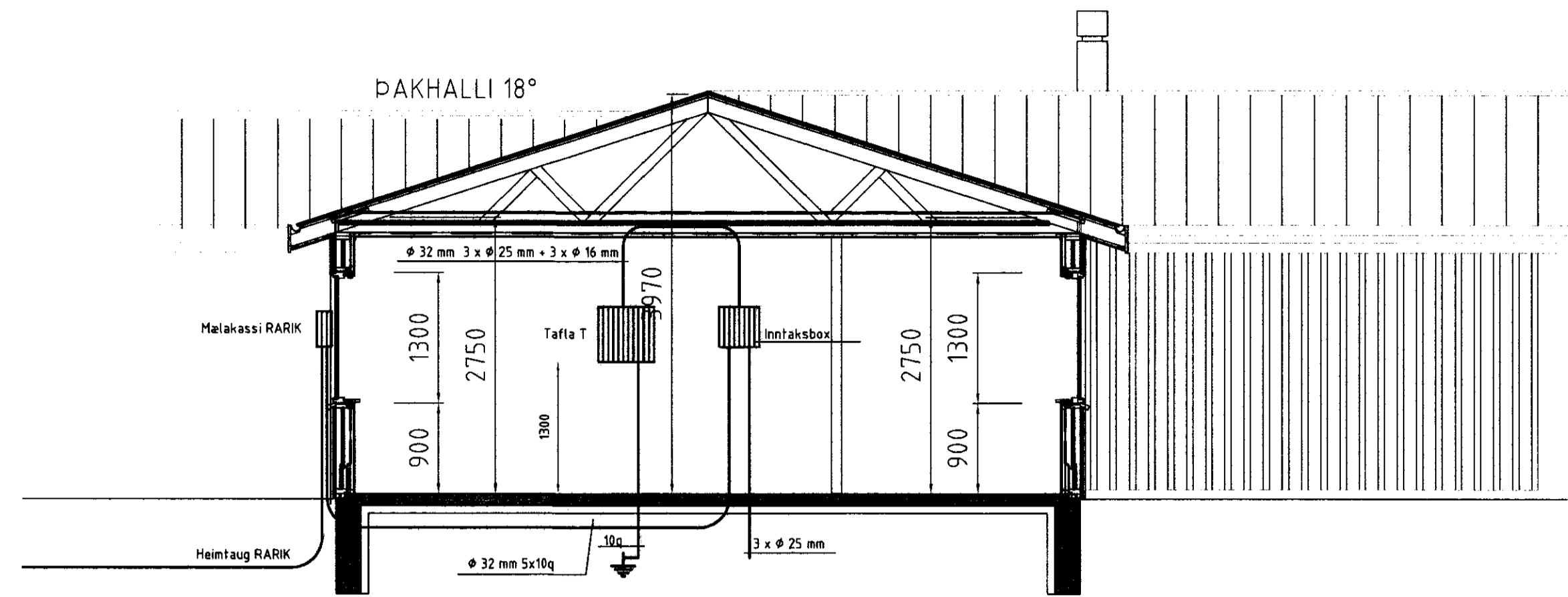
SNEIÐMYND A-A
