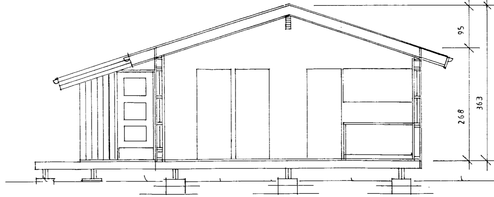
SNÍÐ A-A
