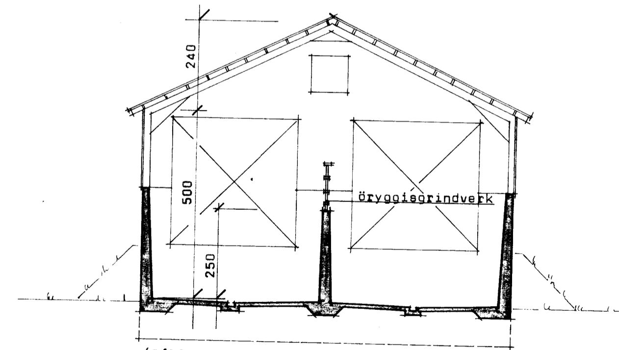
Snið A-A
