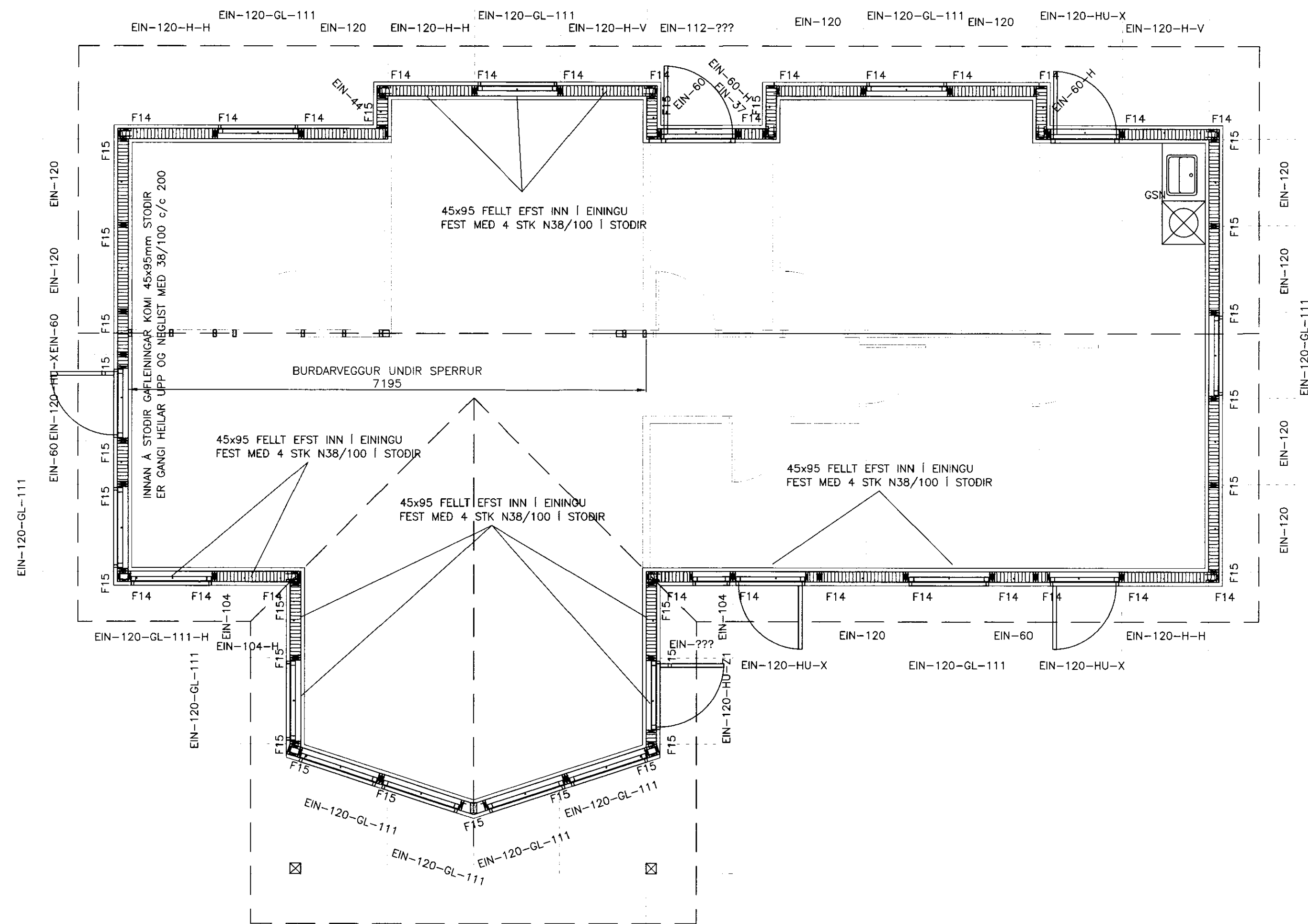
VEGGJAPLAN MKV. 1:50
