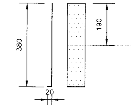
FESTIJÁRN F7 & F7- MKV. 1:10 F7 = 2 Stk. F7- = 1 Stk. BMF-GATAPLATA 2x80x400, BEYGT Í ENDA. NEGLING: 10 STK. KS40/40 Í GÓLFBITA. STEYPT Í SÖKKUL.
