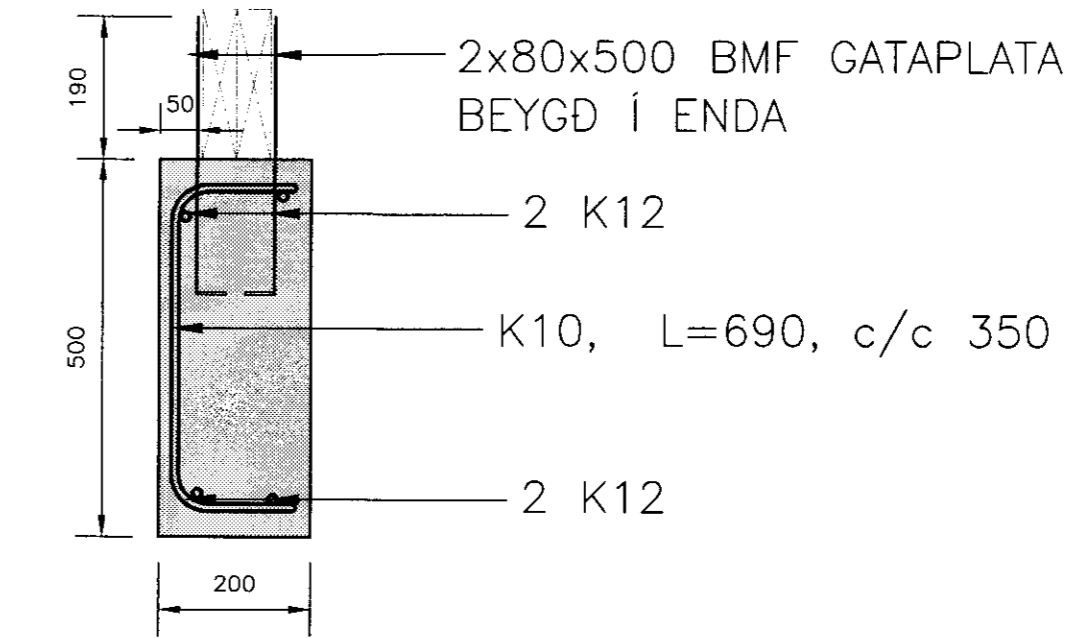
SNID Í SÖKKULVEGG MKV. 1:10
