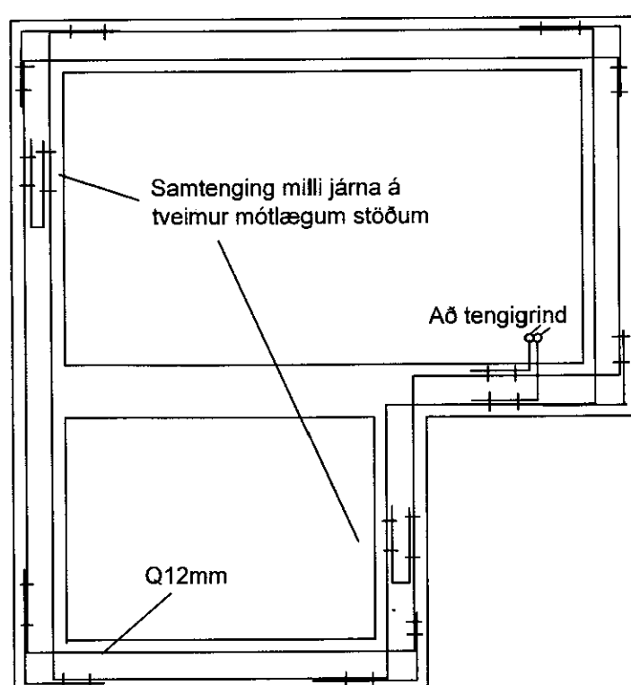
SÖKKULSKAUT Dæmigerður frágangur
