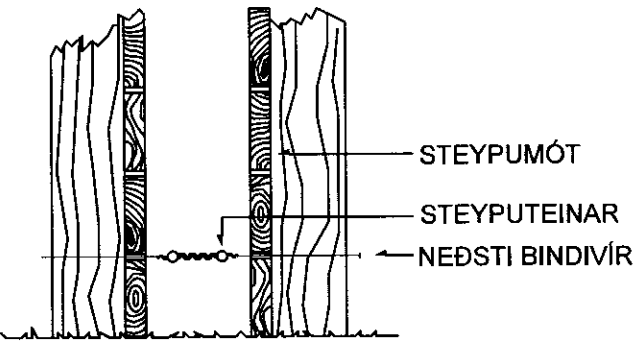
SNIB Í STEYPUMÓT
