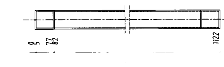
b 2 RHS 80x5 2 stk. skali 1:10
