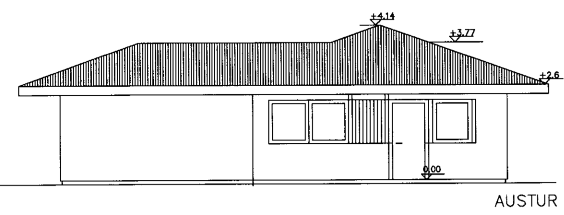
Íbúðarhús hliðar 1:100
