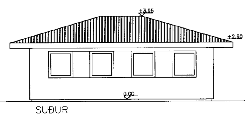
Bílskúr hliðar 1:100
