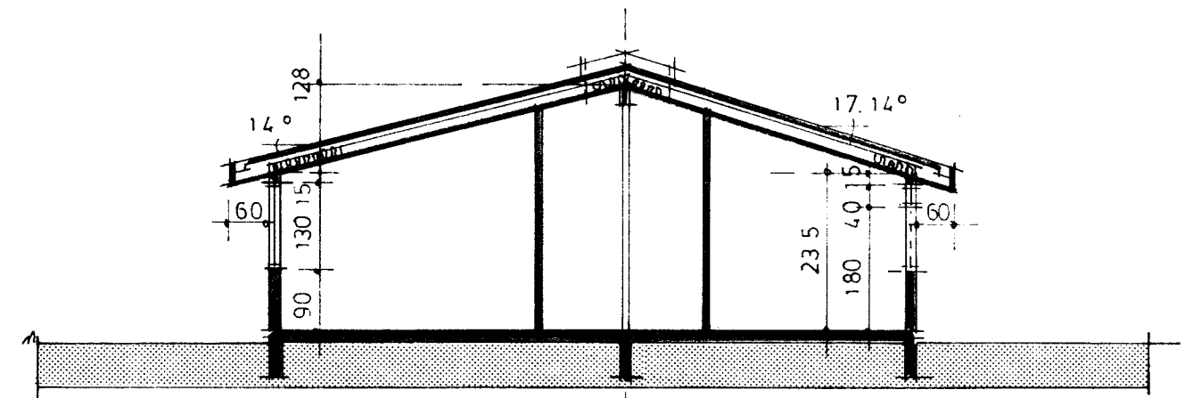
SNID A-A
