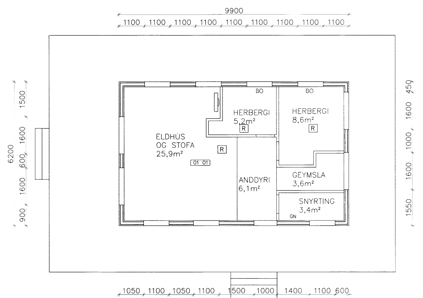
GRUNNMYND 1:100
