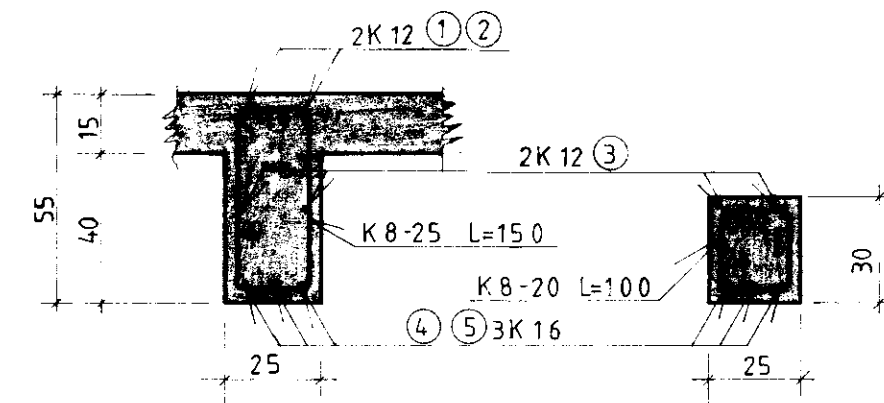
Snid B-B M=1:20 Snid A-A
