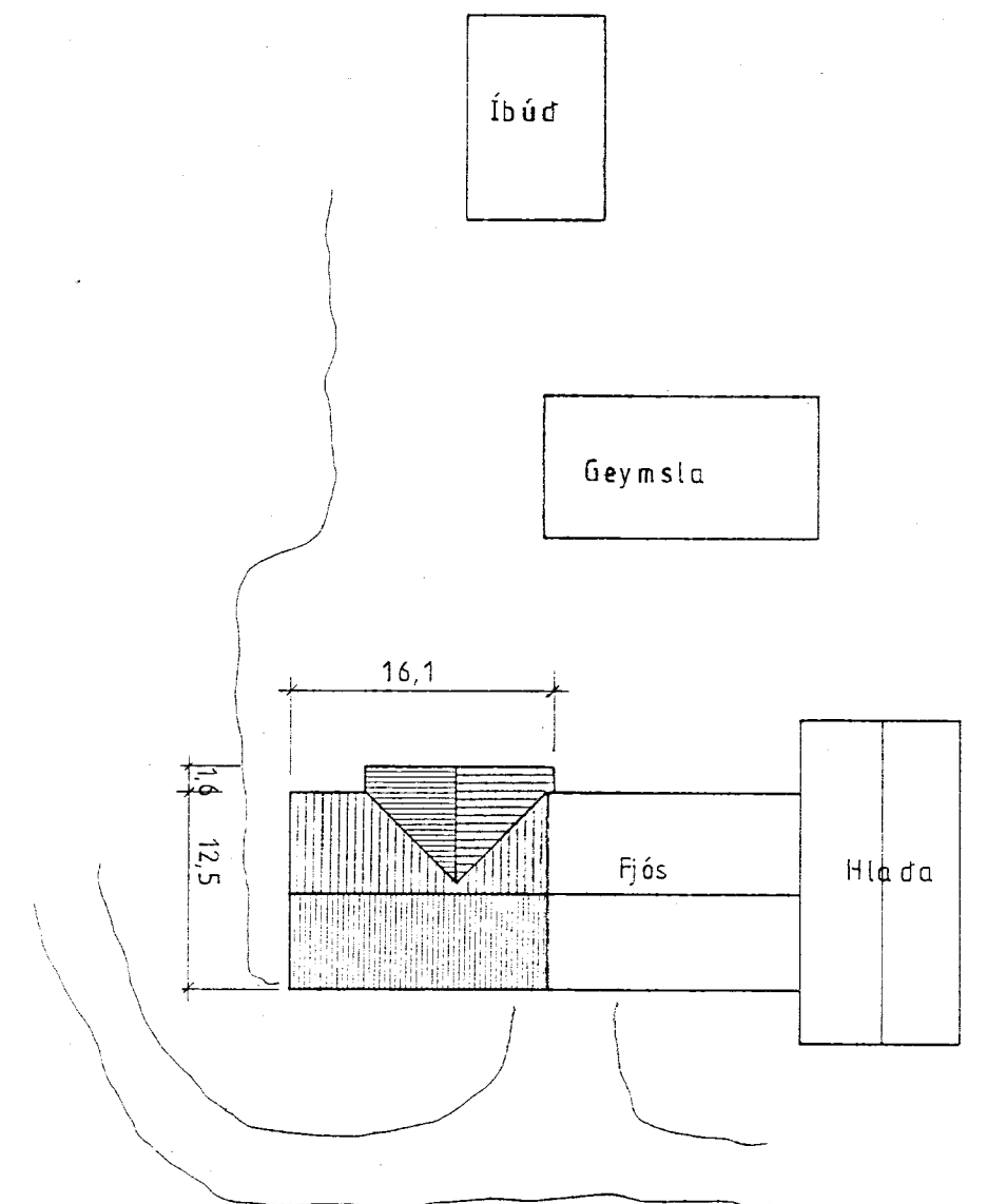
Afstöðumynd M=1:500
