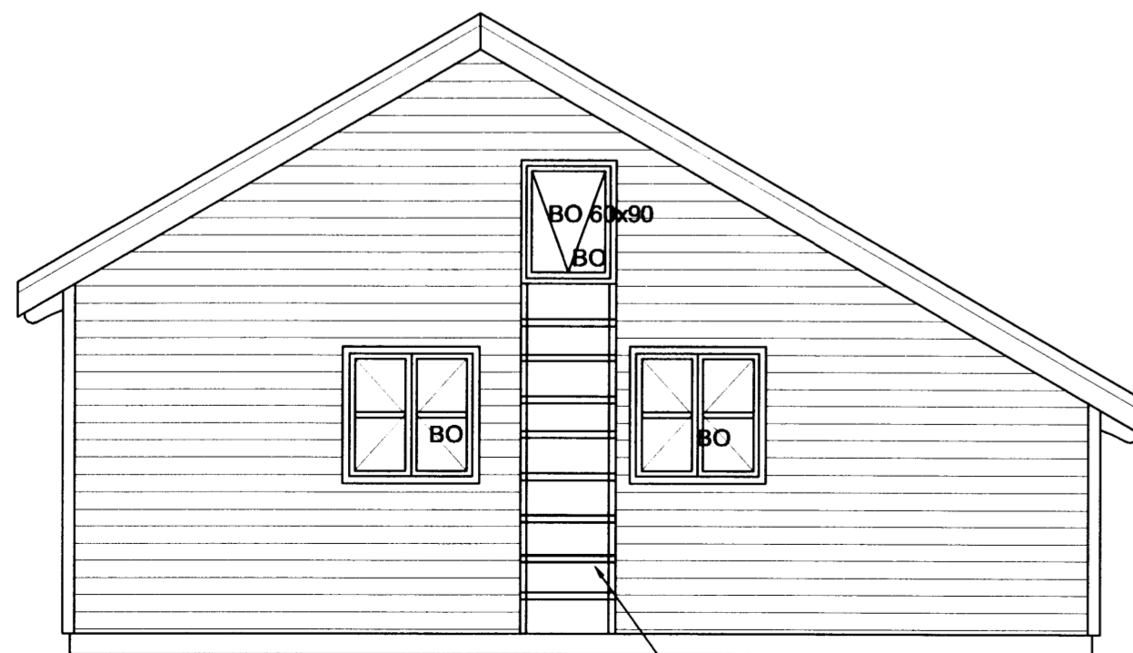
ÚTLIT NORÐUR, MKV. 1:50
