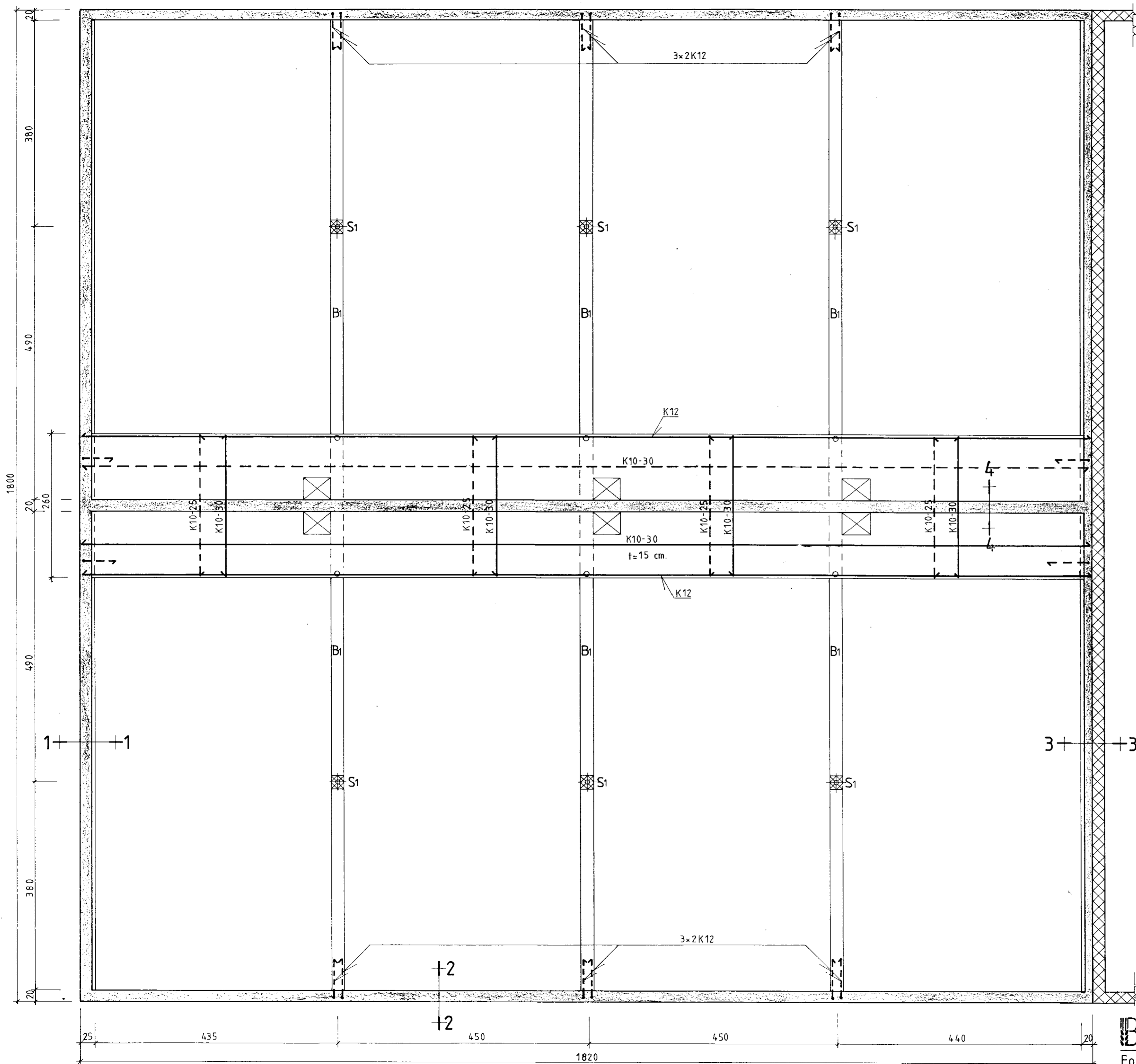
Fjárhúsgólf M=1:50
