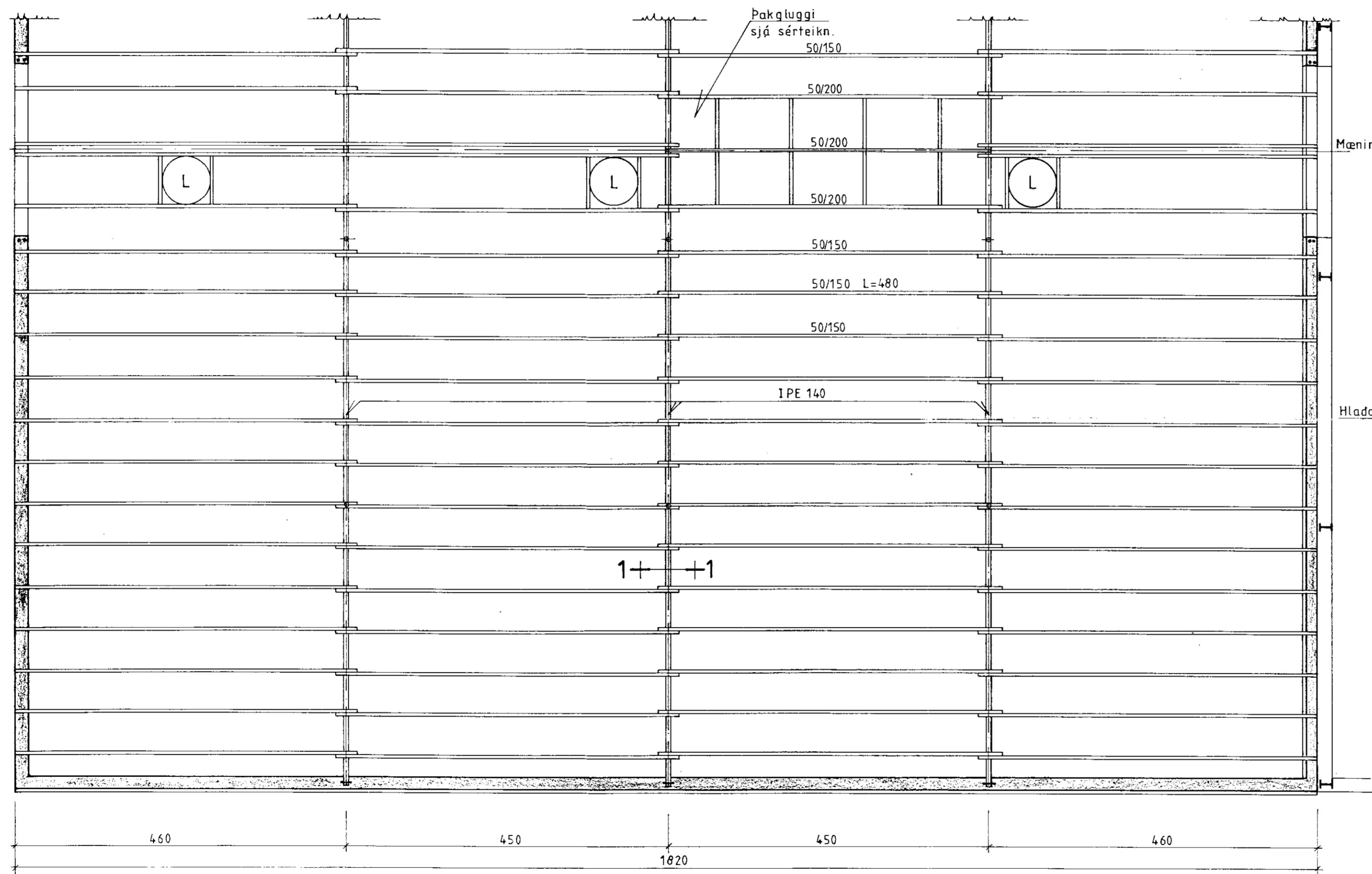
Pak grunnmynd M=1:50
