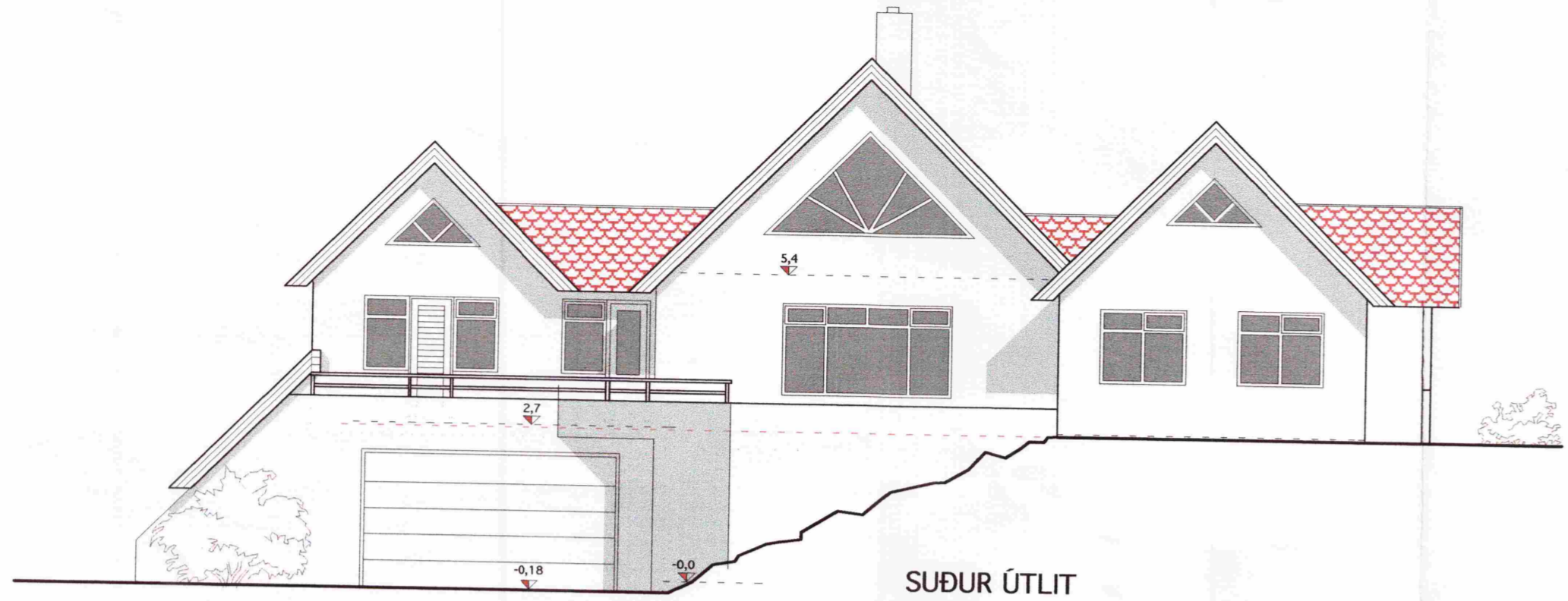
SUÐUR ÚTLIT
