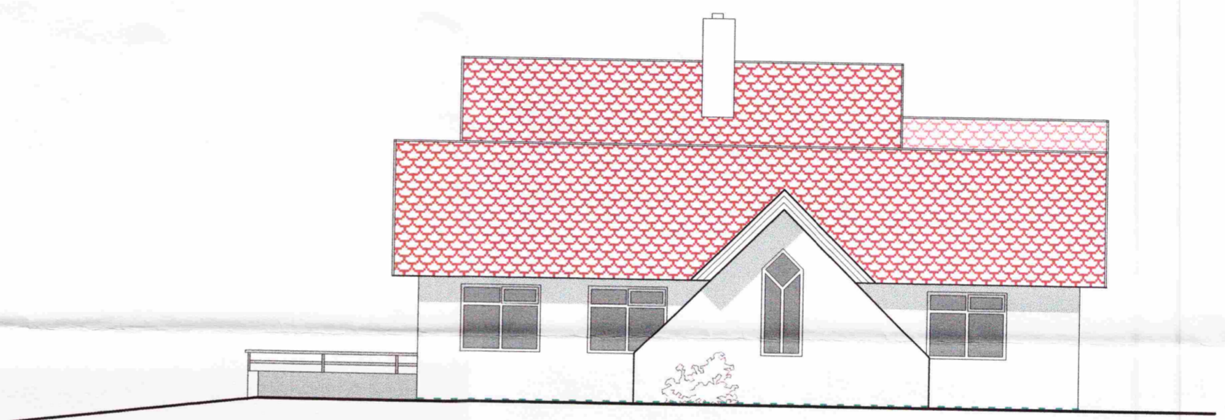
AUSTUR ÚTLIT
