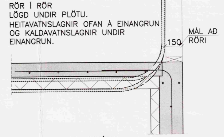
STADSETNING STÚTA VID ÚTVEGG OG UNDIR PLÖTU Mkv. 1:20
