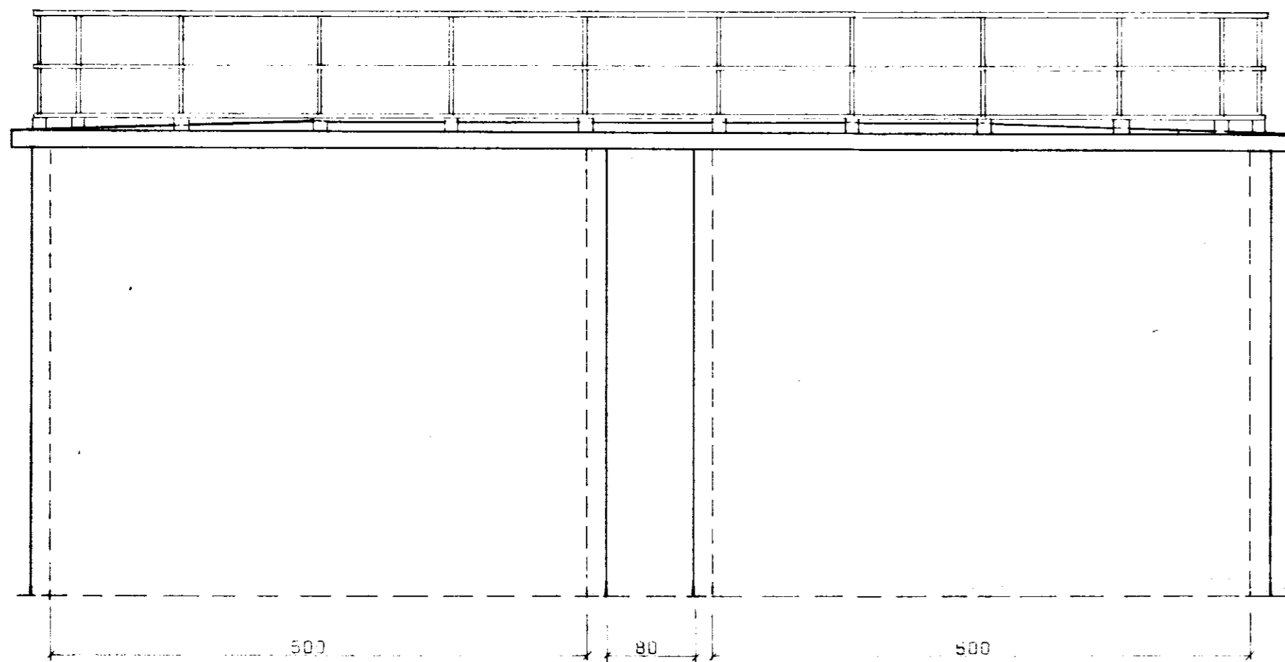
ÞAKPLATA M=1:50
