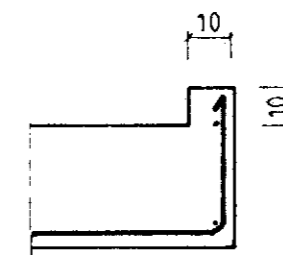
ÞAKLÚGA M=1:10
