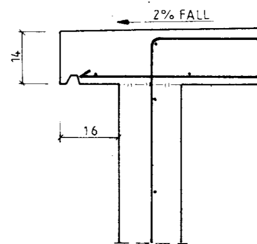
ÞAKBRÚN M=1:10
