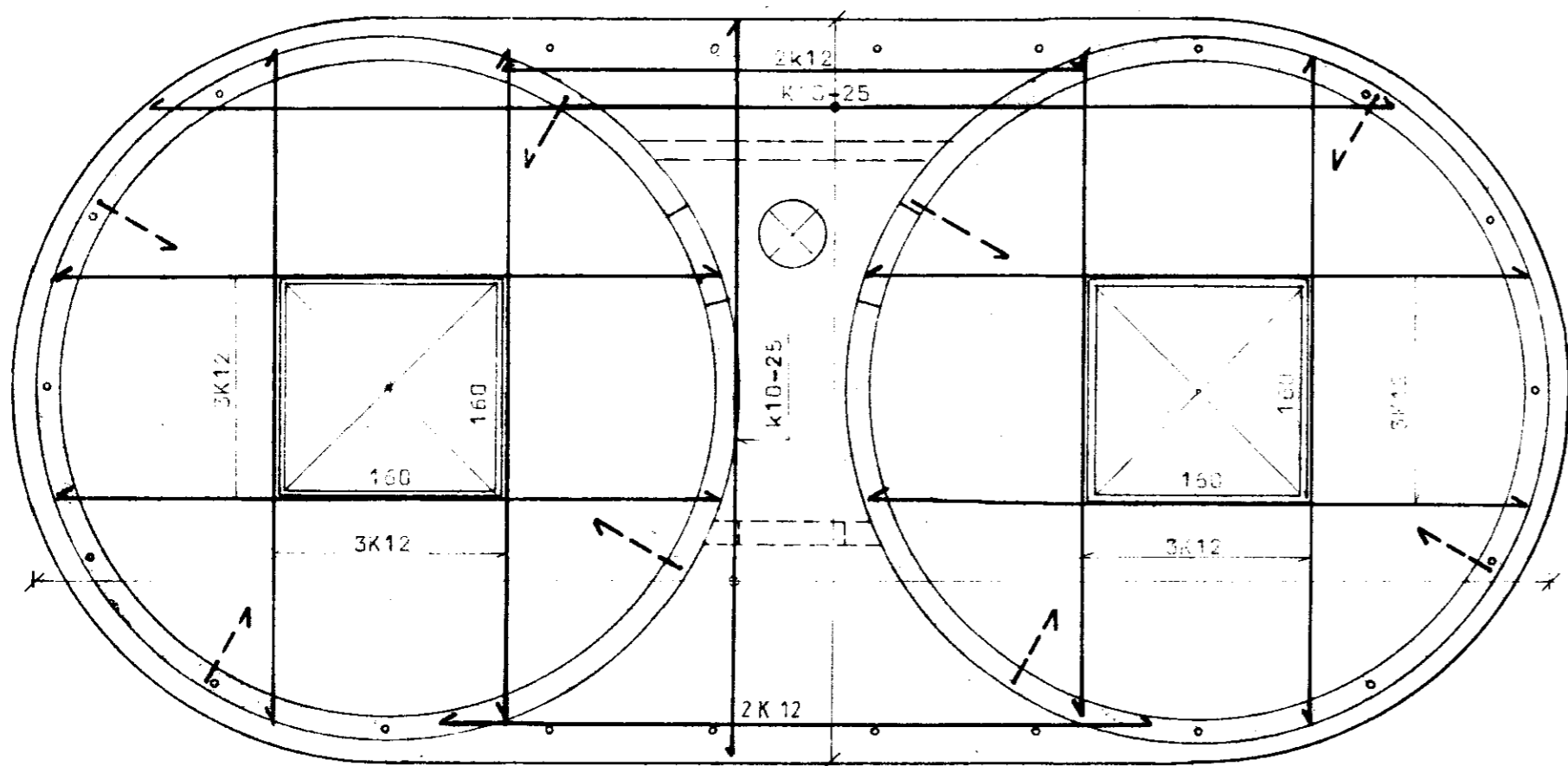
ÞAKPLATA M=1:50
