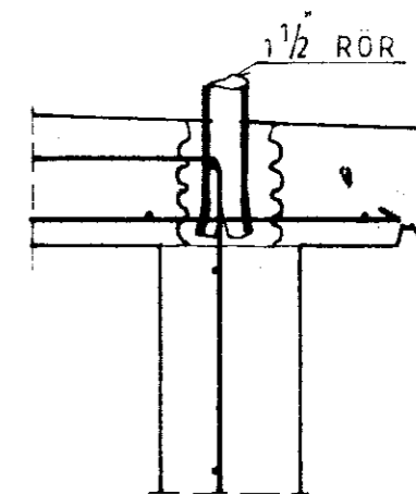
HANDRÍÐSSTÓÐ M=1:10
