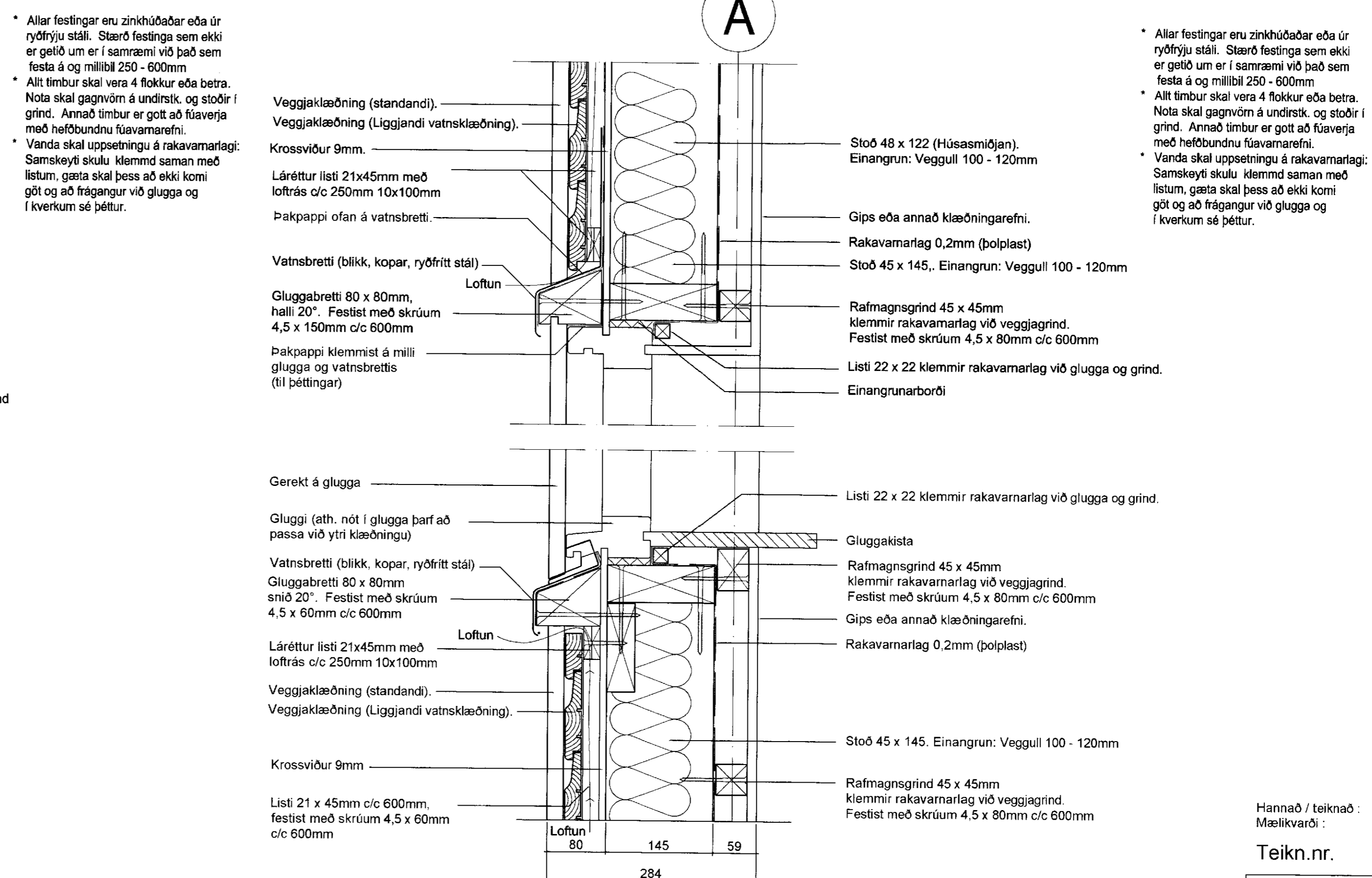
(31)5,1 Útveggur með glugga: Lóðrétt snið.
