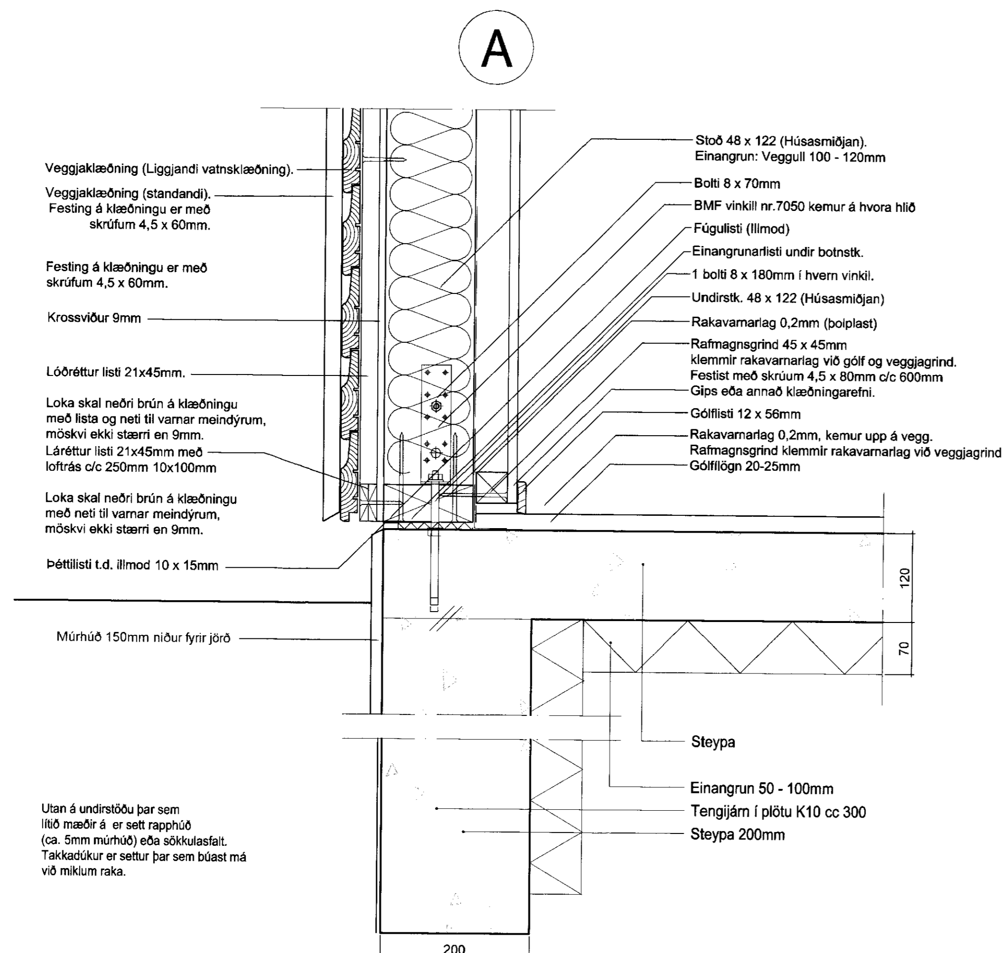
(21)5,5 Útveggur með glugga: Lóðrétt snið.
