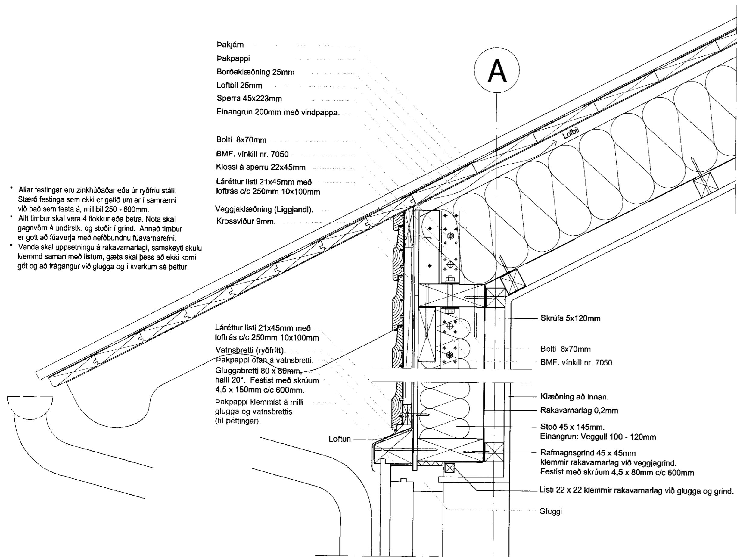
(27) 5,1 Pakfótur: Útveggjklæðning kemur upp í þakklæðningu.
