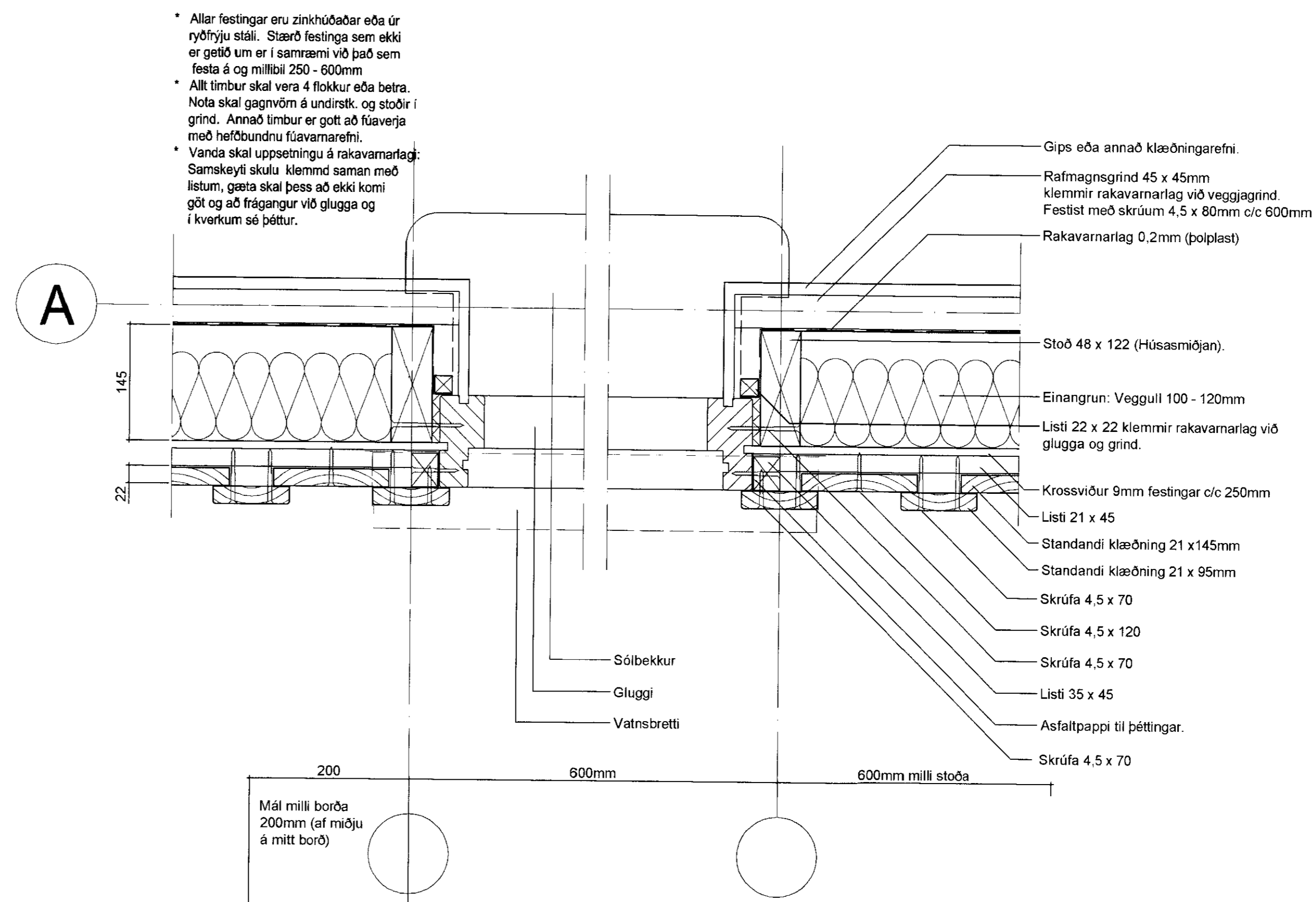
(31)5,2 Útveggur með glugga: Lárétt mynd.
