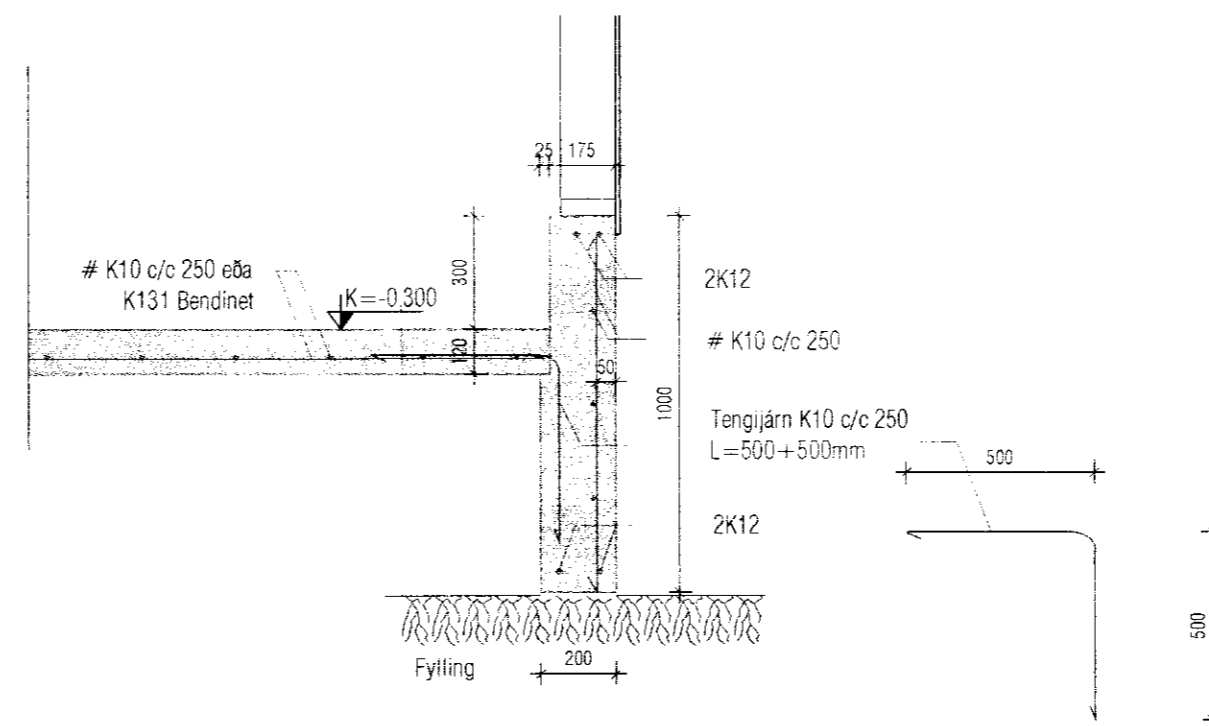
Mkv 1:20 B-B B01
