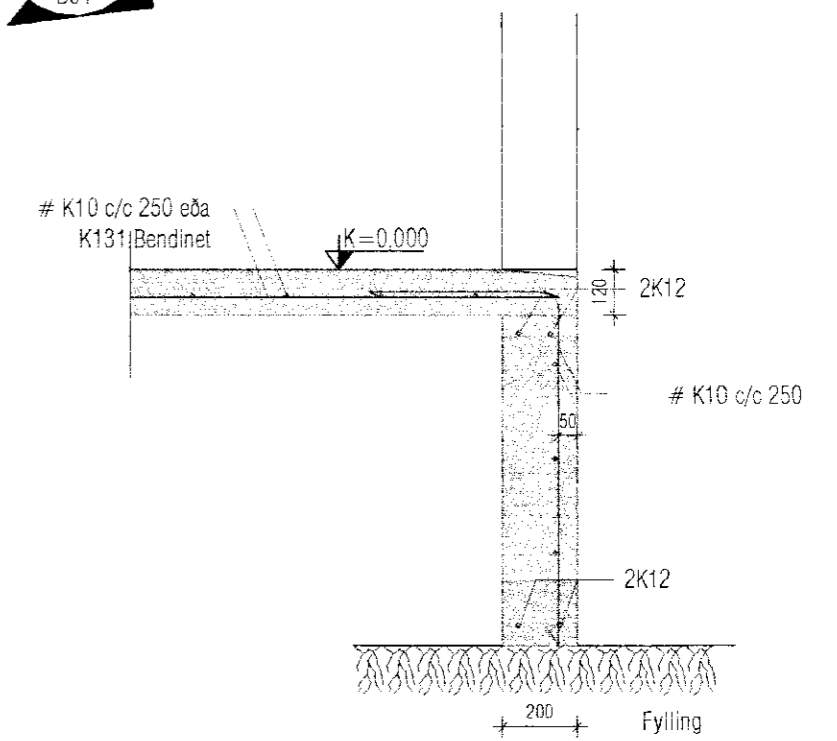
Mkv 1:20 C-C B01
