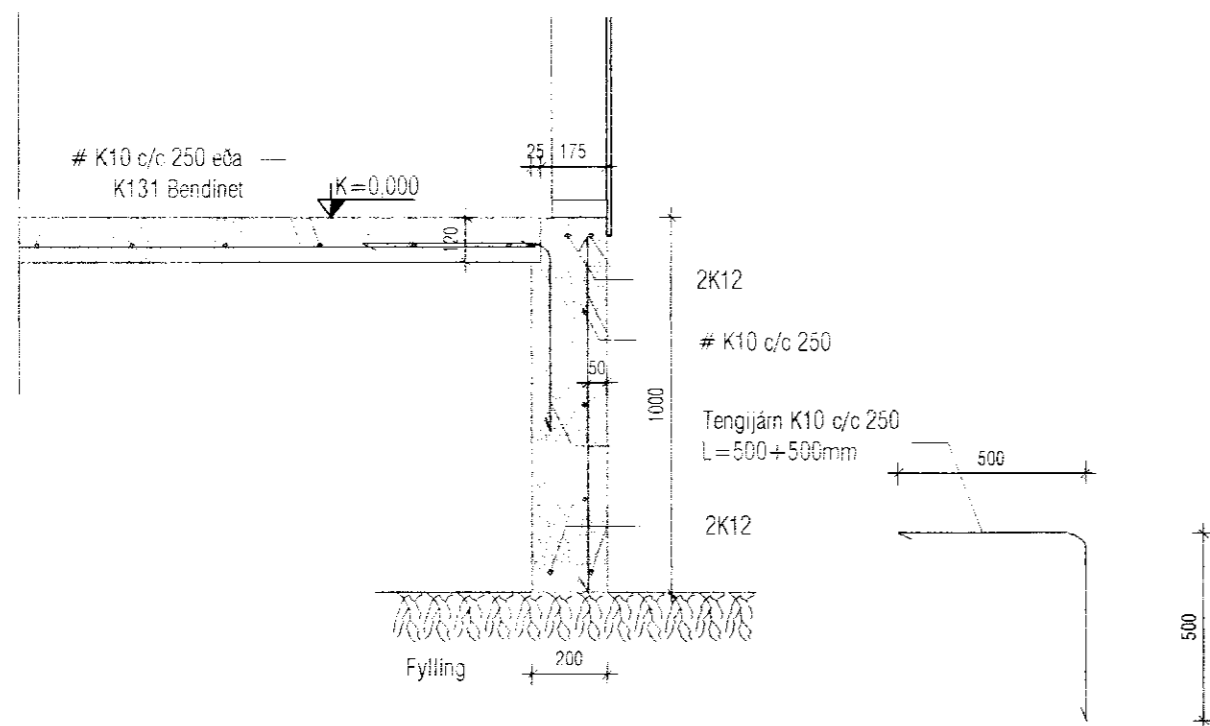
Mkv 1:20 A-A B01
