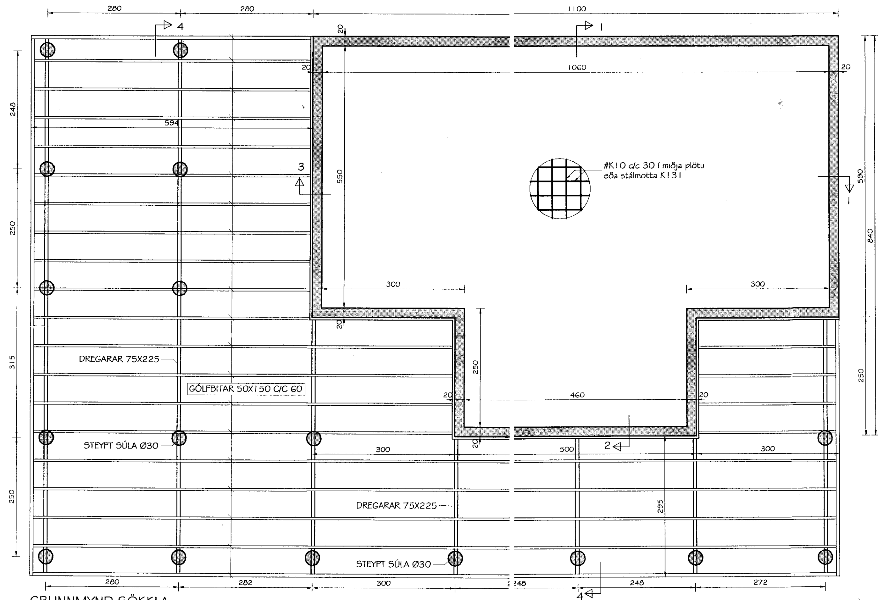
GRUNNMYND SÖKKLA mkv. 1:50
