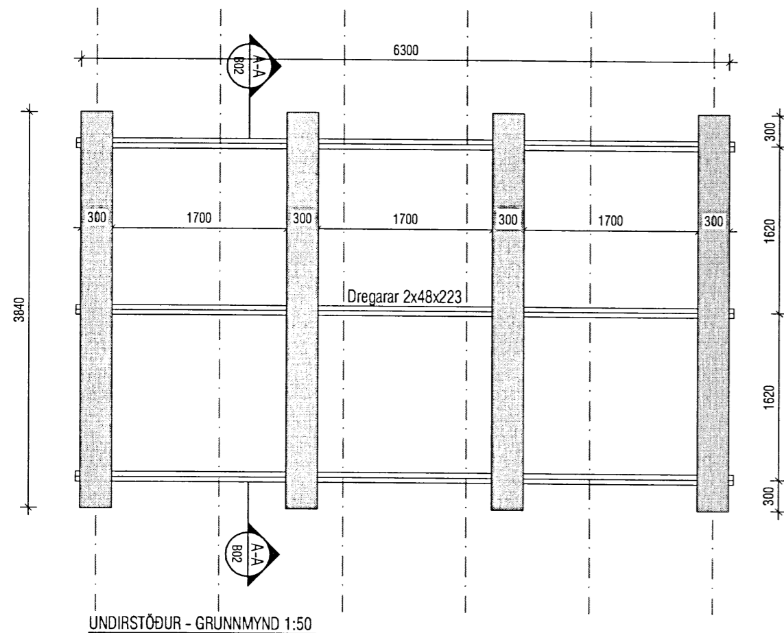
UNDIRSTÖÐUR - GRUNNMYND 1:50
