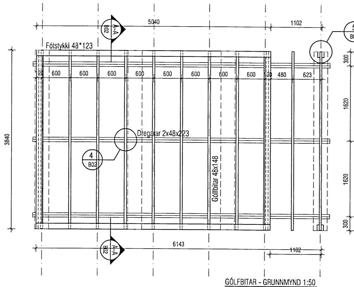
GÓLFBITAR - GRUNNMYND 1:50
