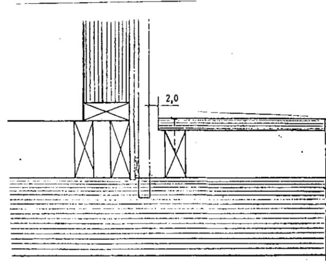
Snid D-D
