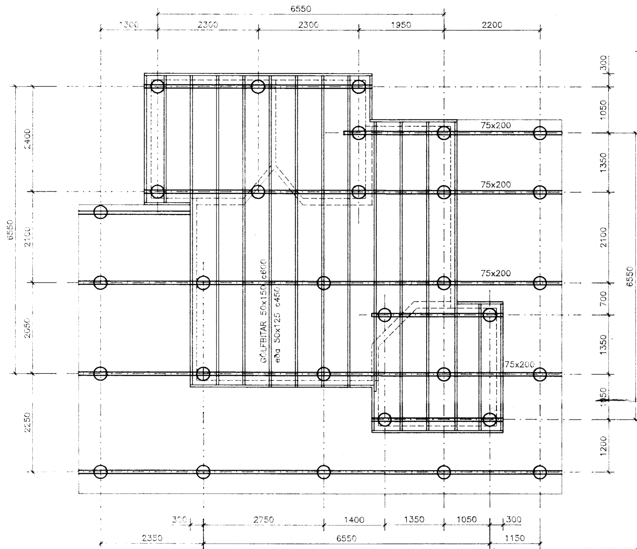
UNDIRSTÖÐUR – GRUNNMYND 1:50
