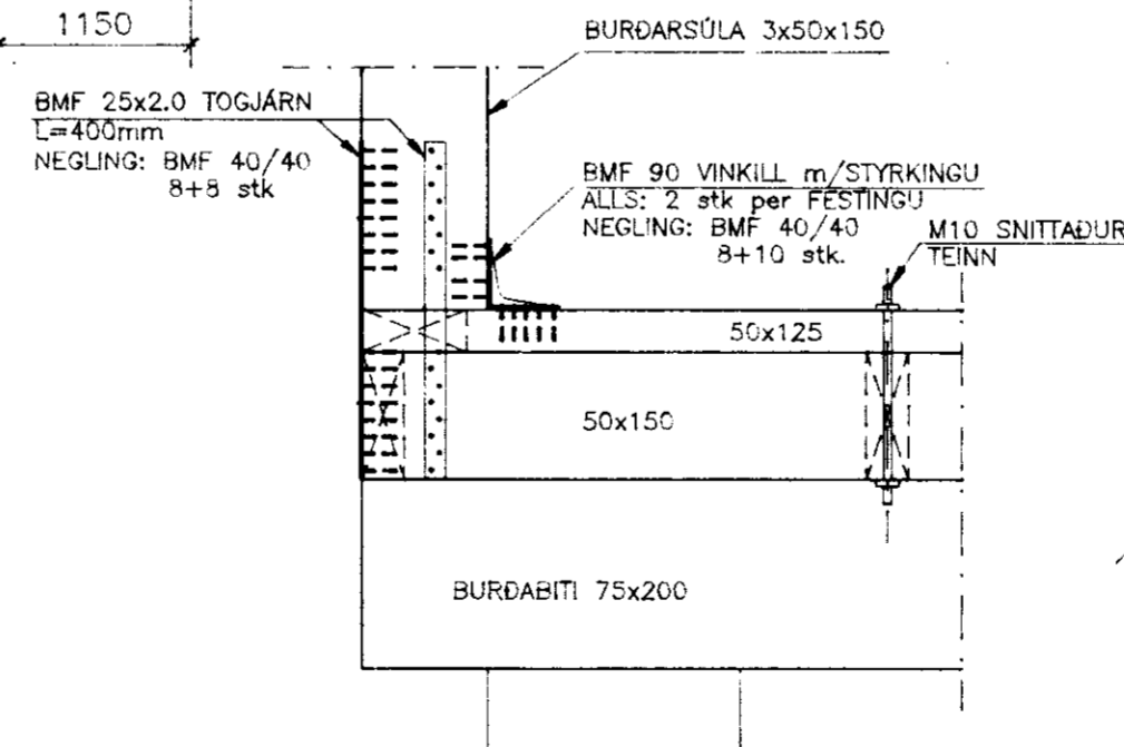
B FESTING SÚLU VIÐ GÖLFBITA 1:10
