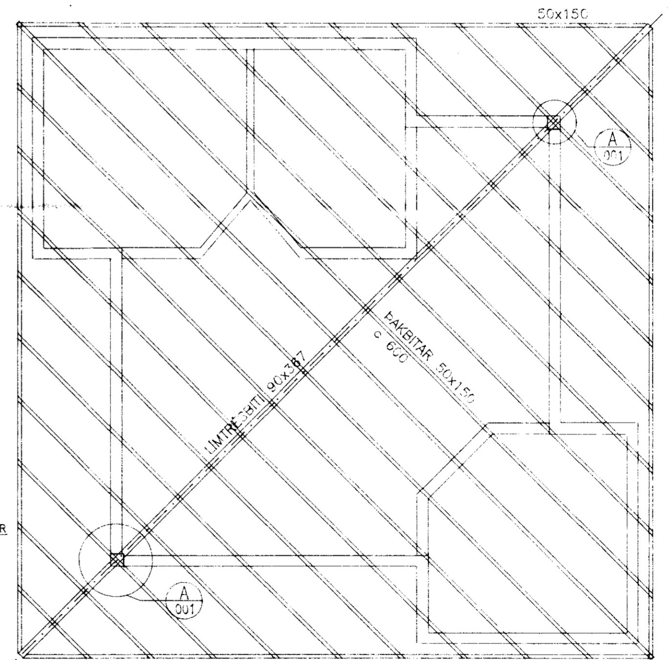
ÞAKVIRKI – GRUNNMYND 1:50
