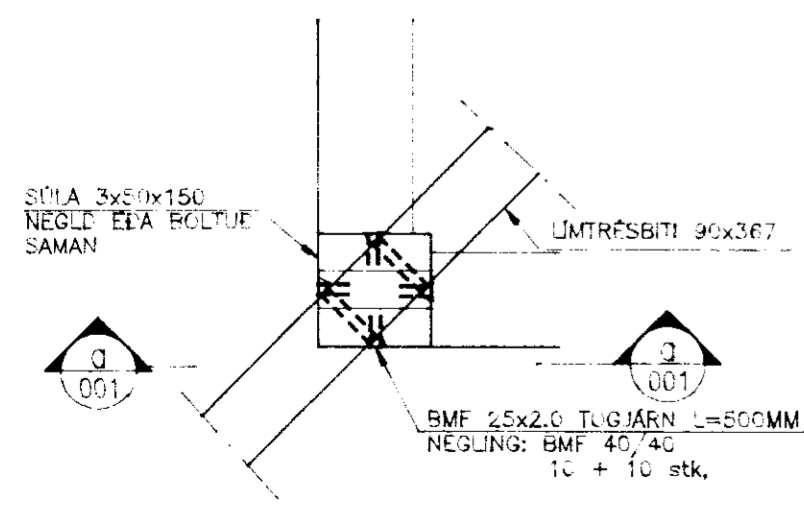
A FESTING LIMTRÉSBITA VIÐ SÚLU 1:10
