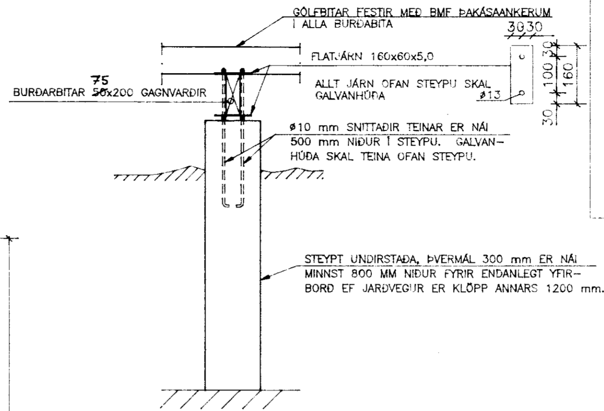
FRÁGANGUR VIÐ UNDIRSTÖÐU 1:20
