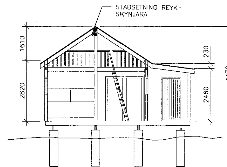
SNID A-A 1:100
