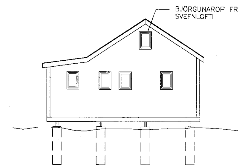
AUSTUR 1:100
