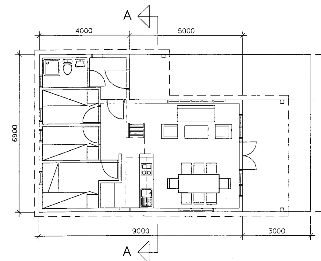
GRUNNMYND 1:100
