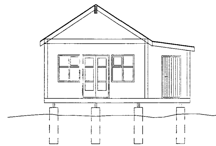
VESTUR 1:100
