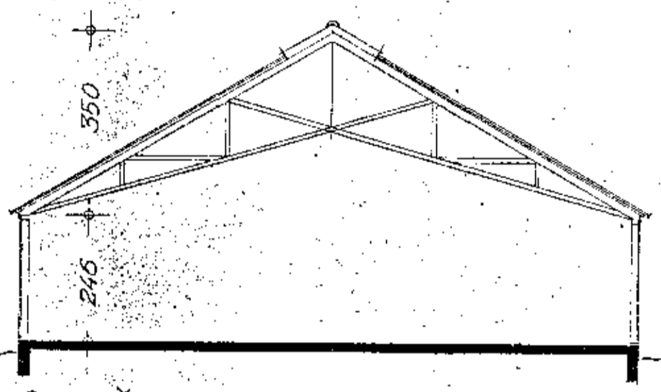
Sneiðing
