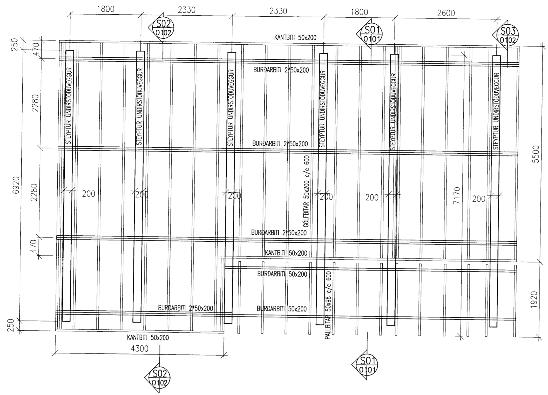
GRUNNMYND SÖKKULL OG GÓLFBITAR, 1:50
