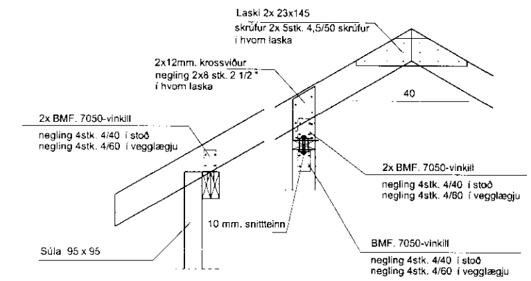
SNID D-D 1:20
