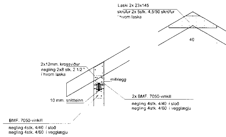
SNID B-B 1:20
