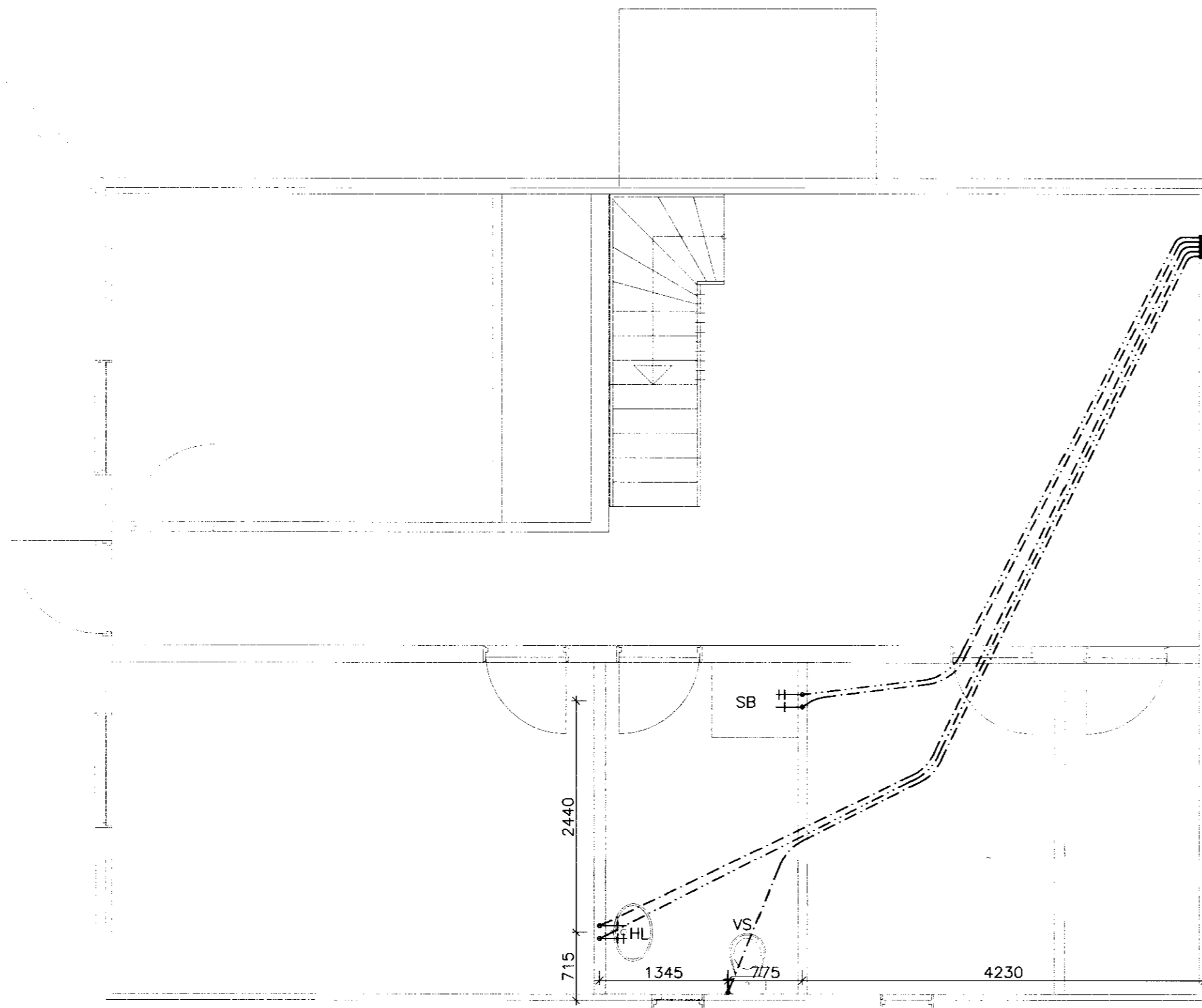
KJALLARI GRUNNMYND NEYSLUVATNSLAGNA 1:50
