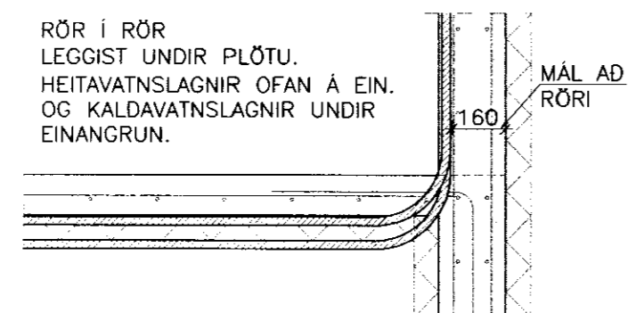
STADSETNING STÚTA Í ÚTVEGG OG UNDIR PLÖTU Í KJALLARA Mkv. 1:20
