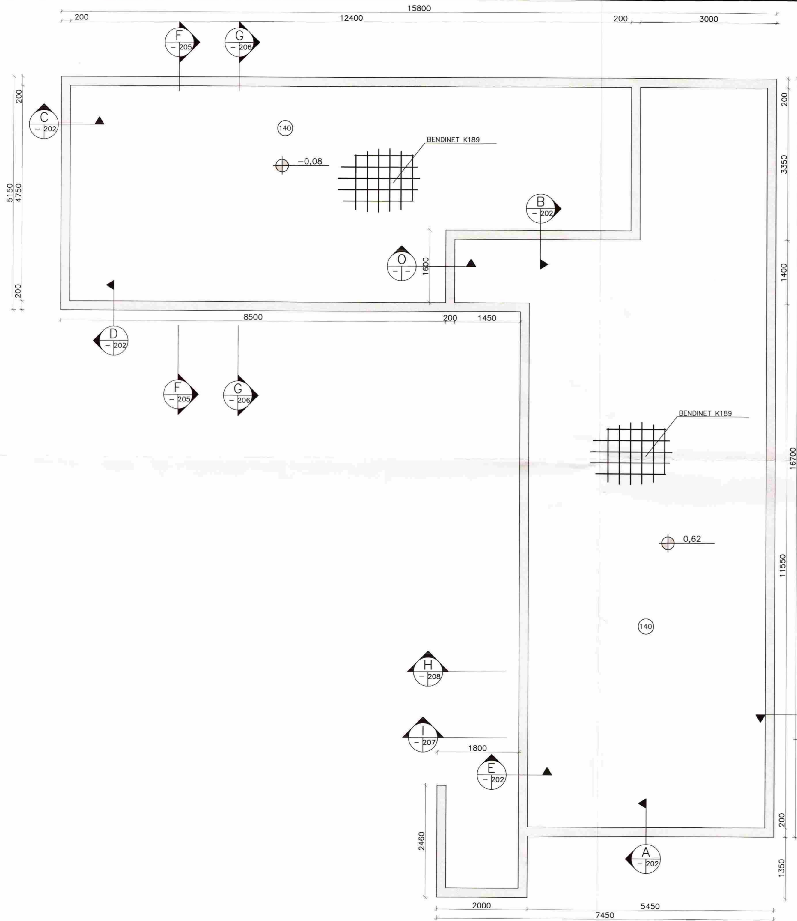
GRUNNMYND SÖKKLA OG BOTNPLÖTU 1:50
