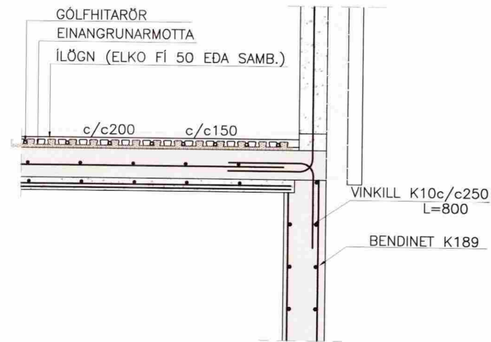
FRÁGANGUR GÓLFGEISLA Á 2.HÆÐ 1:20
