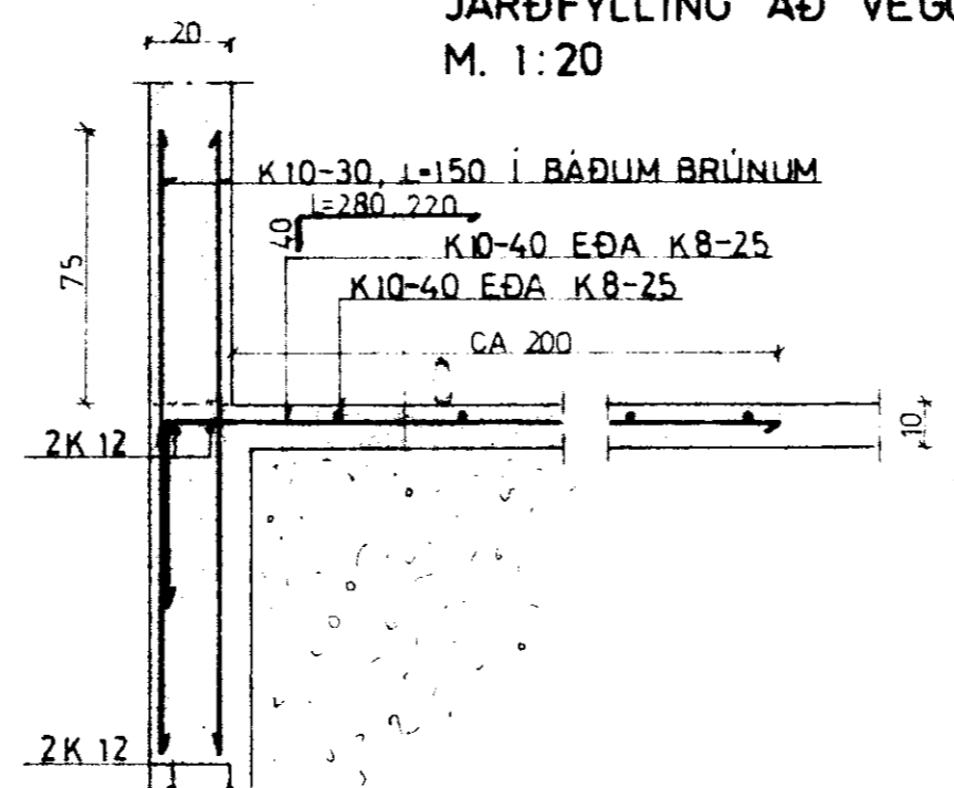
SNID 4-4 HÁIR SÖKKLAR LITIL JARÐFYLLING AÐ VEGG M. 1:20
